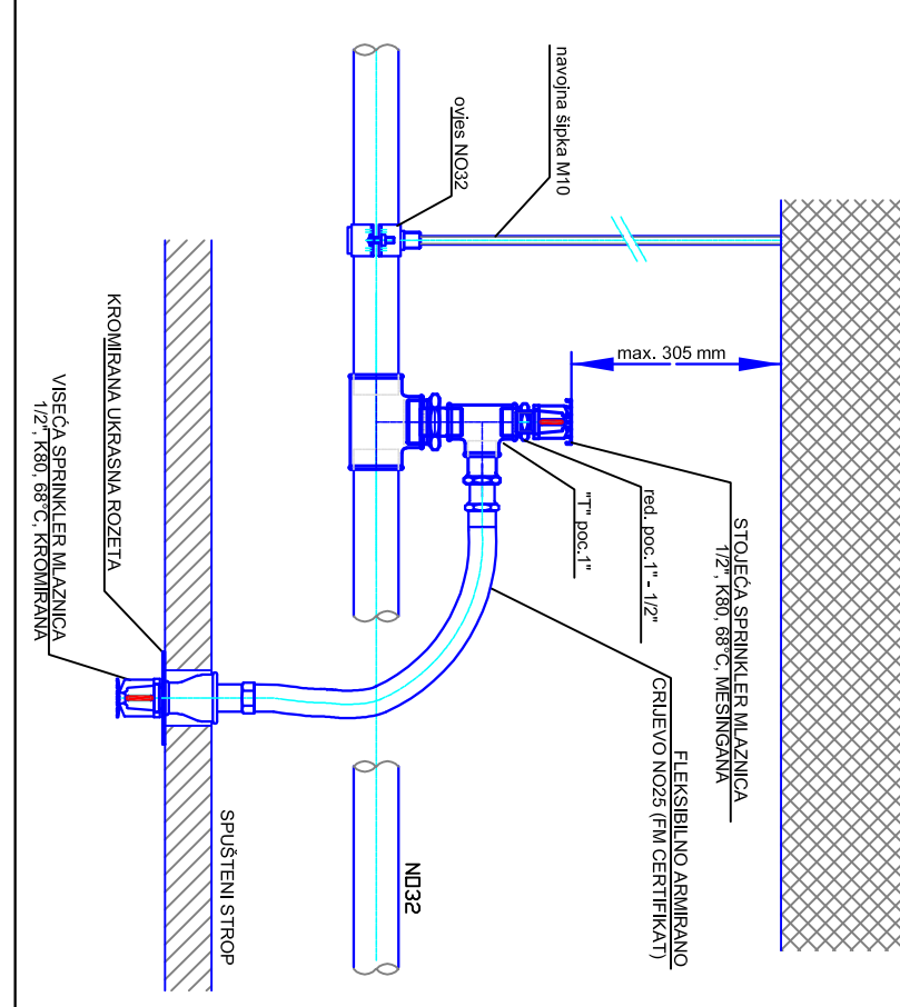
Detalj 5 Detalj montaže mlaznice i sprinkler
