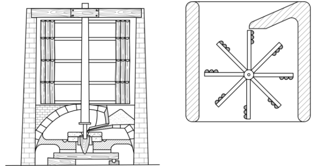
Slika 2. Perzijska vjetrenjača
