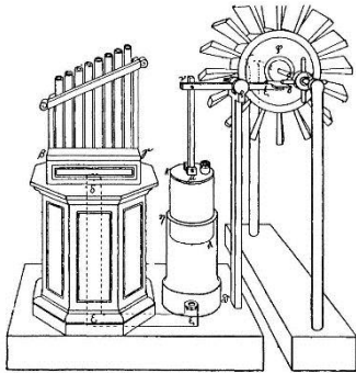
Slika 1. Heronova vjetrenjača
