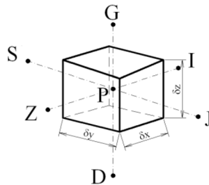
Sl. 3.1. Kontrolni volumen s prikazanim čvorovima susjednih kontrolnih volumena
