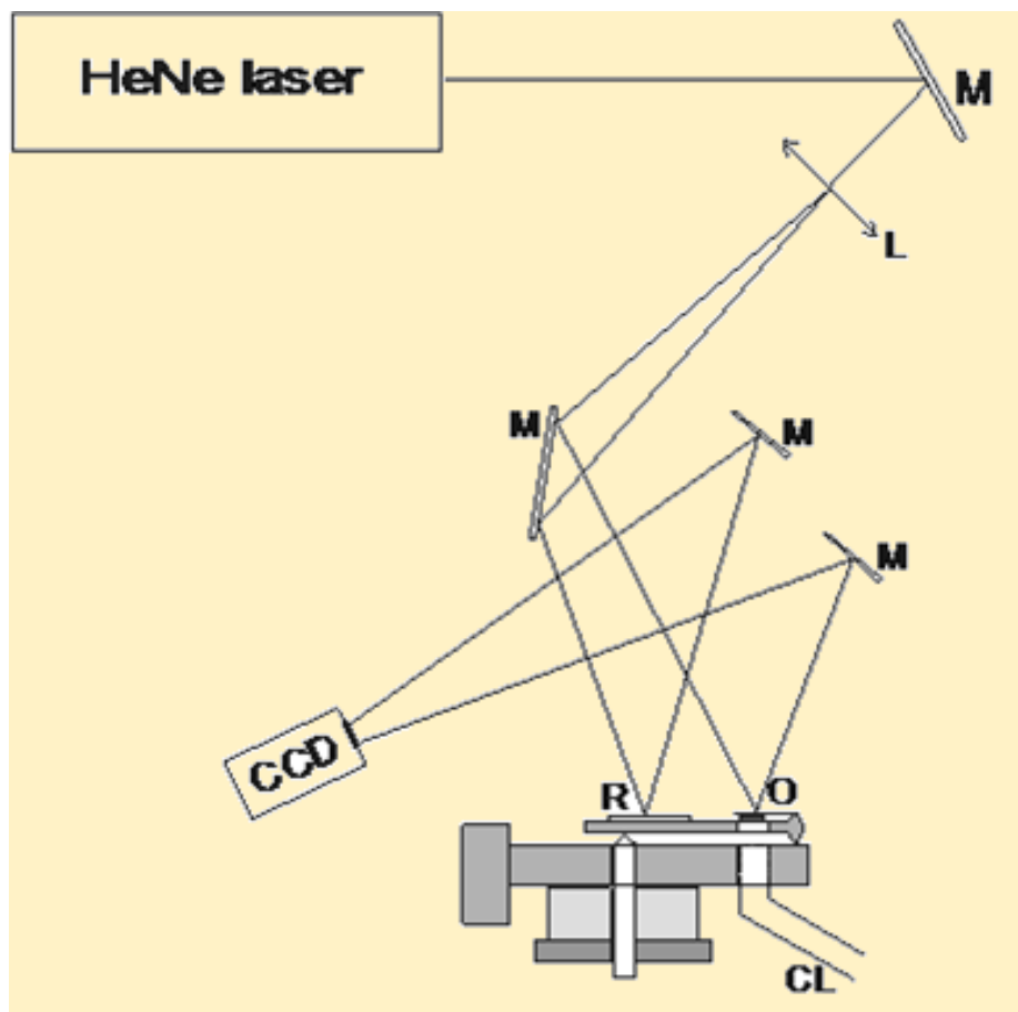
Slika 8. Eksperimentalni postav
