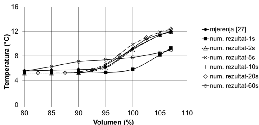
Slika 4.35. Usporedba izlaznog profila temperature num. proračuna s podacima mjerenja za različite vremenske korake kod procesa pražnjenja ( Re=3778 , Fr=0,14 [27])
