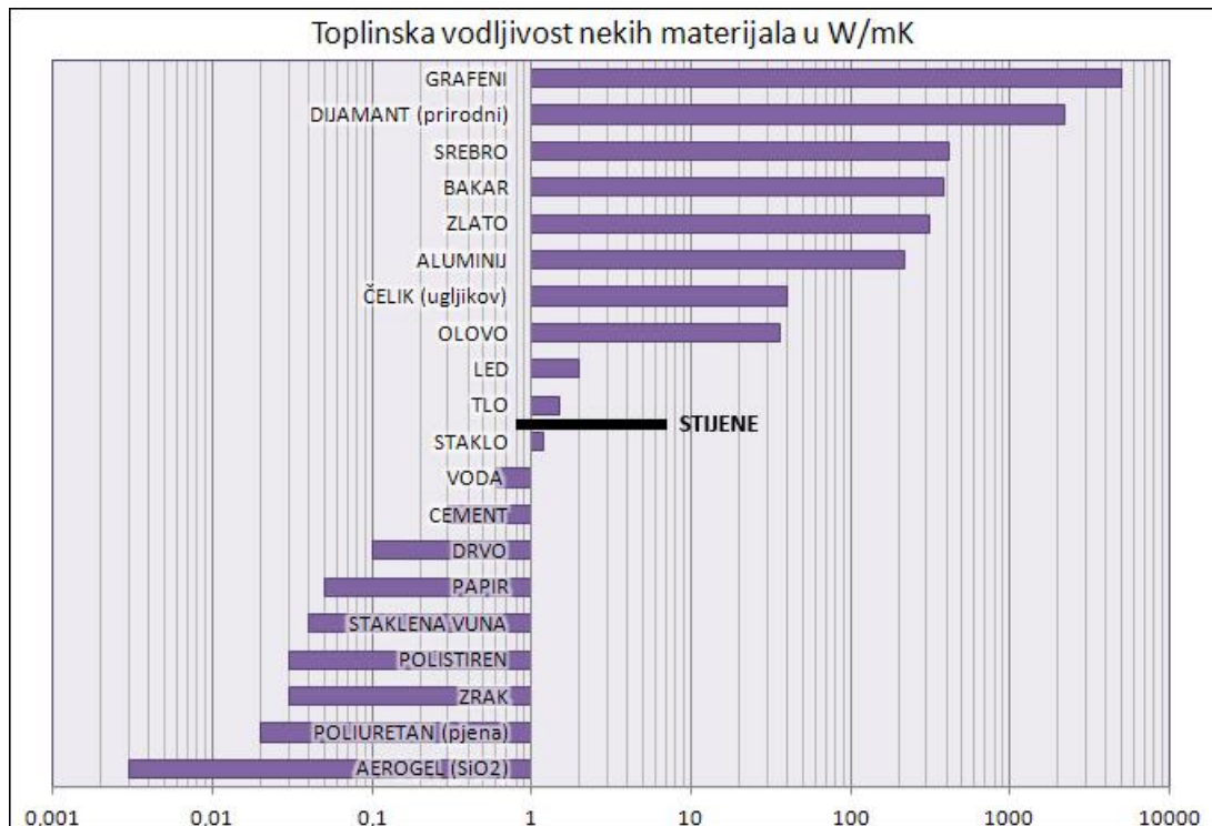
Slika 5.8. Toplinske vodljivosti nekih materijala (izvor: Beardsmore & Cull, 2001)
