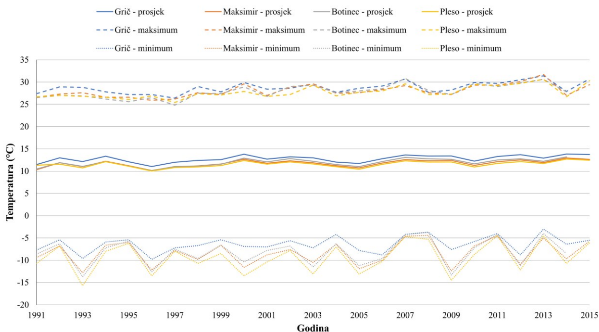
Slika 5.9. Prosječne, maksimalne i minimalne godišnje vrijednosti srednjih dnevni temperatura zraka
