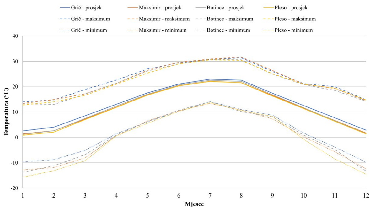
Slika 5.10. Prosječne, maksimalne i minimalne mjesečne vrijednosti srednjih dnevni temperatura
