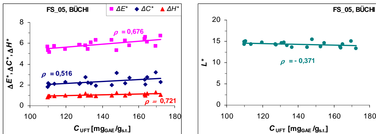
Slika 4.41. Ovisnost ukupne promjene boje ( \Delta E^* ), promjene kromatičnosti ( \Delta C^* ), promjene tona boje ( \Delta H^* ) i svjetline ( L^* ) ekstrakata sjemenki grožđa FS_05 o masenom udjelu ukupnih fenolnih tvari – C_{UFT} (podaci za ekstrakte dobivene pomoću 50%-tnog etanola nakon ekstrakcije u vremenu trajanja od 20 do 200 minuta uz primjenu četiri metode ekstrakcije univerzalnog sustava Büchi - Soxhlet standard, kontinuirana ekstrakcija, Soxhlet topli i vruća ekstrakcija)
