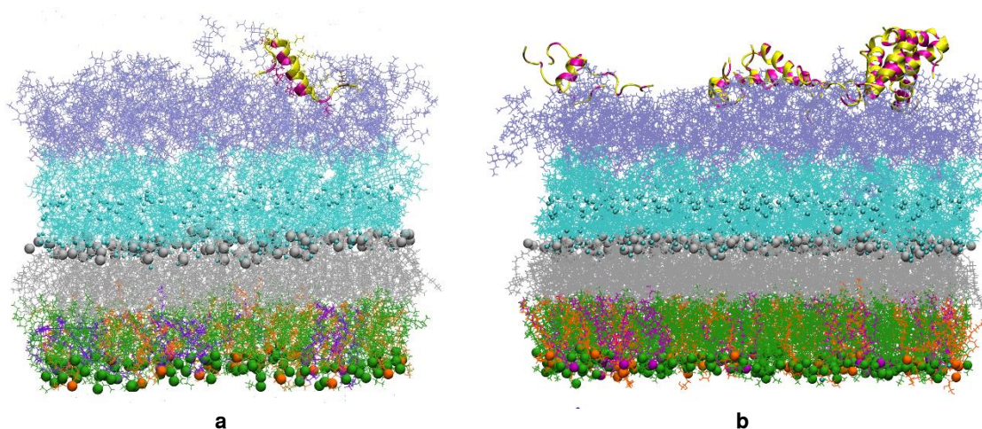
Slika 42 Vanjske membrane Gram-negativnih bakterija s 2 O-antigena (glatka) u interakciji s jednim peptidom ( a ) ili dvanaest peptida ( b ) nakon 500 ns odnosno 400 ns. Peptidi su inicijalno postavljeni u otopinu 2 nm iznad gornje površine membrane. Svi peptidi uglavnom ostaju vezani za membranu tijekom vremena simulacije. PVPE lipidi su zeleni, PVPG lipidi su narančasti, PVCL2 je ljubičast, a lipid A je siv, a svi su predstavljeni štapićima i kuglicama. Područje jezgre LPS-a predstavljeno je tirkiznim linijama, neutralizirajući \text{Ca}^{2+} ioni u području jezgre predstavljeni su tirkiznim kuglicama, a 2 O-antigena predstavljena su ljubičastim linijama. Peptidi su prikazani kao vrpce, s polarnim i nabijenim ostacima u žutoj i hidrofobnim ostacima u magenta boji. Molekule vode i ioni iz otopine nisu prikazani radi preglednosti.
