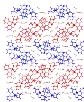
11b·3CH 3 OH
