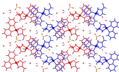
11a·6H 2 O
