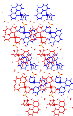
10a·6H 2 O
