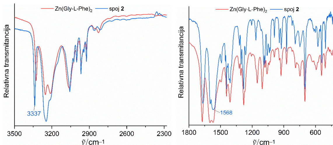
Slika 31. IR spektri \text{Zn}(\text{Gly-L-Phe})_2 i spoja 2 u području 3500\text{--}2300\text{ cm}^{-1} (lijevo) i 1800\text{--}400\text{ cm}^{-1} (desno).
