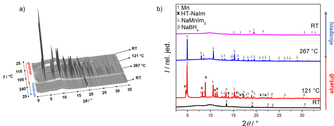
Slika IX. a) Difrakcijske slike uzorka 6D1 prikupljene tijekom grijanja u temperaturnom intervalu 25–295 °C te tijekom ciklusa hlađenja do 25 °C b) Fazni sastav uzorka 6D1 na 25, 121, 267 te 25 °C u hlađenju. Difrakcijske linije visokotemperaturnog polimorfa \text{NaIm} označene su s \times , \text{NaMnIm}_3 s \lambda , \text{Mn} s \tau , dok je \text{NaBH}_4 označen s \beta .
