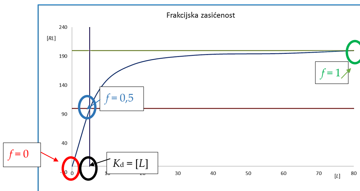
Slika 15. Frakcijska zasićenost, f_i u ovisnosti o koncentraciji liganda [L] pri konstantnoj temperaturi. Vrijednost frakcijskog zasićenja kreće se od 0 (nema interakcija) do 1 (kada su sve molekule receptora vezane s ligandom). Izvor: Prilagođeno prema Kuriyan, Konforti & Wemmer. Molecular Recognition : The Thermodynamics of Binding. Mol. Life 1–58 (2009).
