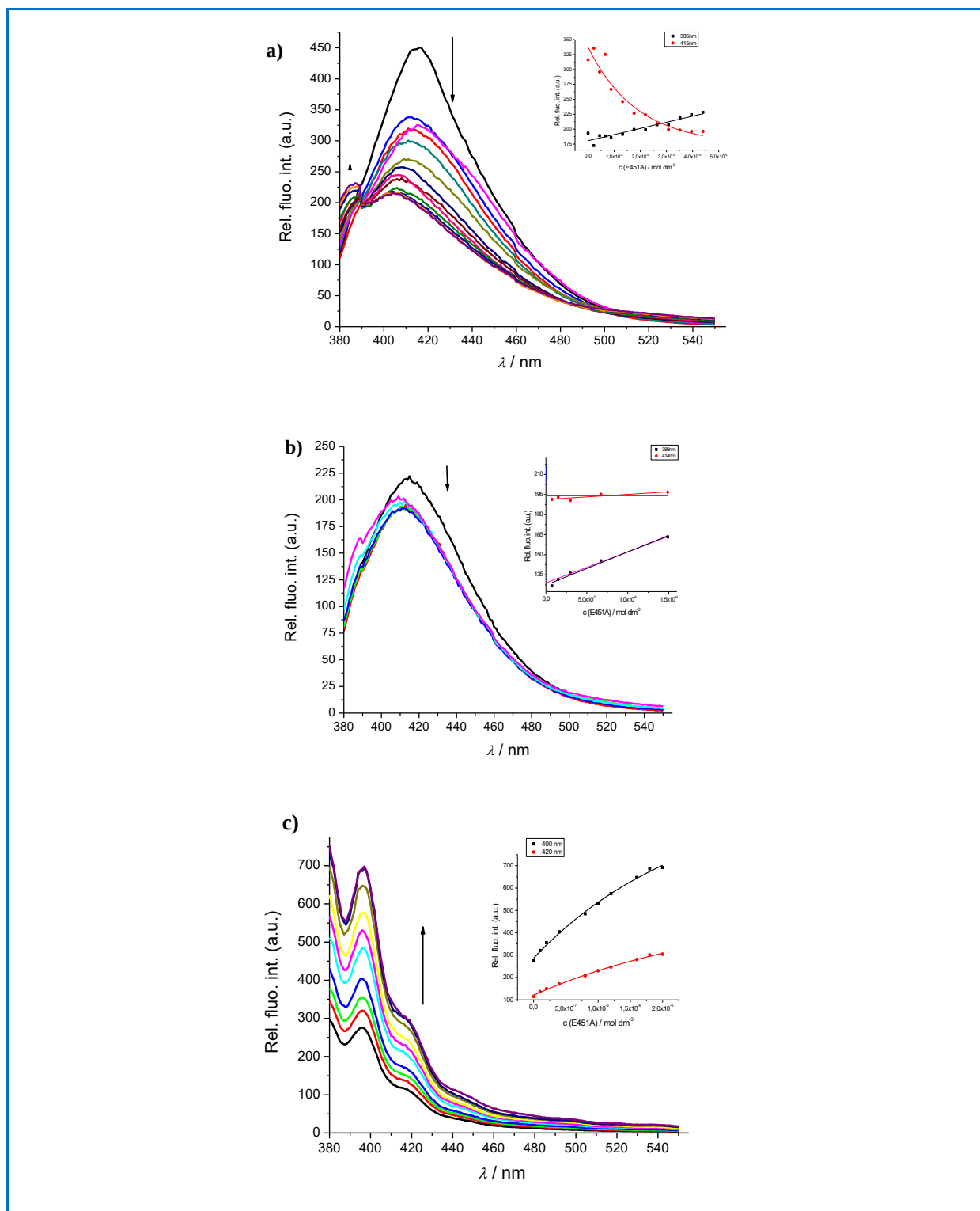
Slika 22. Promjene fluorescencijskih spektara puferških otopina novosintetiziranih spojeva: a) A ; b) B ; c) C ; ( c = 1 \times 10^{-8} mol \text{dm}^{-3} ; pH 7,4; I = 0,05 mol \text{dm}^{-3} ) pri različitim koncentracijama dodanih alikvota ishodišne otopine inaktivnog E451A ( c_0 = 1,8 \times 10^{-4} mol \text{dm}^{-3} ; koncentracijski raspon od \approx 1 \times 10^{-7} mol \text{dm}^{-3} - 4,4 \times 10^{-6} mol \text{dm}^{-3} ) pri 25 °C.
