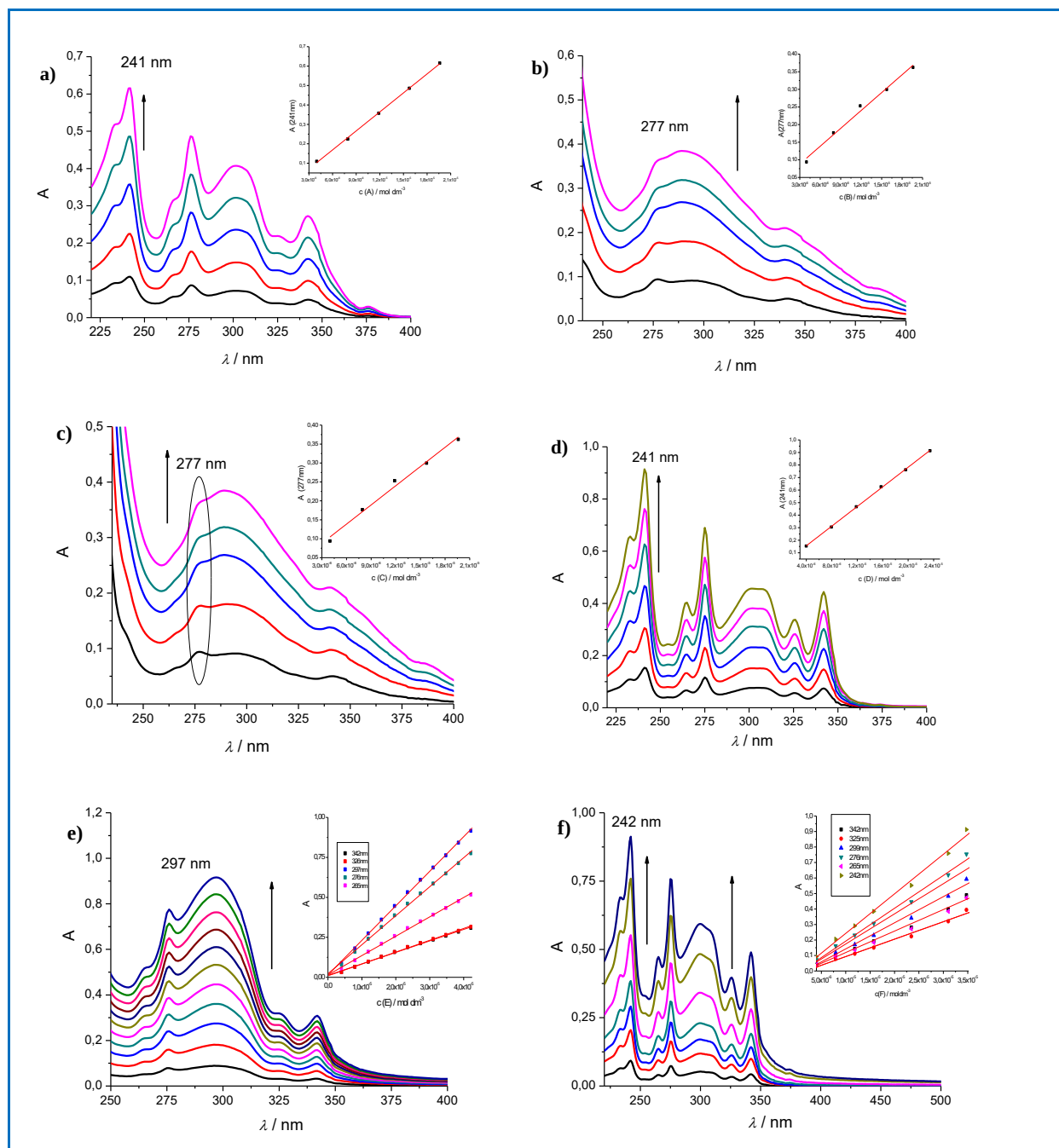
D-Slika 1. Ovisnost UV/Vis spektra o koncentraciji za novოსინთეზირანе спојеве a) A; b) B; c) C; d) D; e) E; f) F. Umetak: Lambert-Beerova linearizacija apsorbancije ( \lambda_{\max} ) u ovisnosti o koncentraciji spoja (puferska otopina natrijeva kakodilata, pH 7, I = 0,05 \text{ mol dm}^{-3} ).
