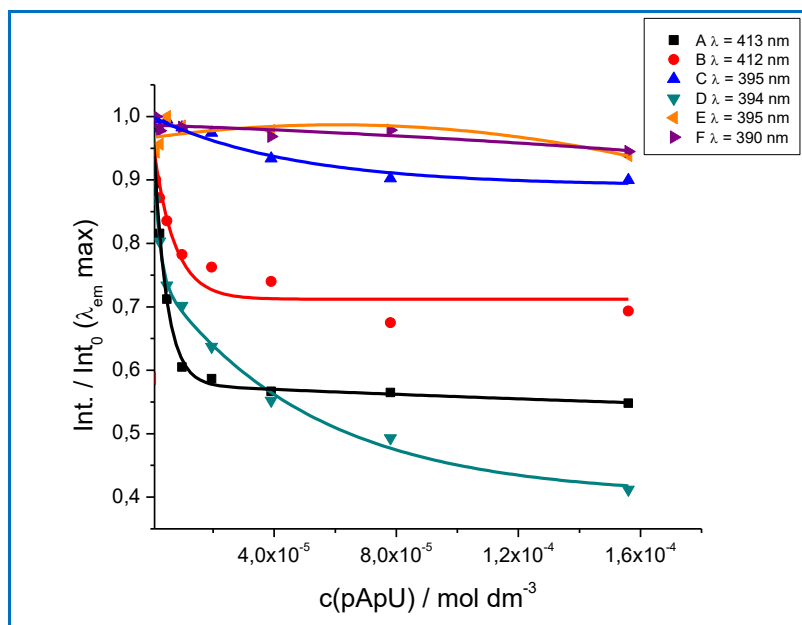
Slika 45. Usporedba rezultata fluorimetrijske titracije novოსინтетизираних спојева A-F ( c = 2 \times 10^{-7} \text{ mol dm}^{-3} , \lambda_{\text{exc}} \approx 342 \text{ nm} ) s pApU, u puferškoj otopini natrijeva kakodilata, pH 7,4, I = 0,05 \text{ mol dm}^{-3} pri 25^\circ \text{C} ; vrijednosti su normalizirane prema polaznom intenzitetu \text{Int}_0 pri emisiji spoja \lambda_{\text{max}} \in [390-415] \text{ nm} .
