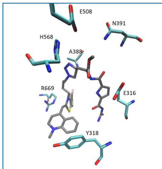
Slika 32. Interakcije CIA -M3 s aminokiselinskim ostacima u aktivnom mjestu hDPP III. Struktura dobivena nakon 200 ns MD simulacija E451A- CIA -M3 kompleksa (prikazani su aminokiselinski ostatci smješeni na udaljenosti manjoj od 4 Å od CIA).
