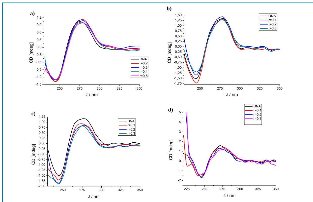
D-Slika 15. Promjene CD spektara otopine ctDNA ( c_{\text{DNA}} = 2 \times 10^{-5} \text{ mol dm}^{-3} ), u puferu natrijeva kakodilata, pri pH 7,4, I = 0,05 \text{ mol dm}^{-3} , pri 25^\circ\text{C} , \lambda_{\text{exc}} = 342 \text{ nm} , slitovi 10 – 10, inkubacijsko vrijeme 0 sekundi, s dodatkom novოსინтетизированог spoja: a) A ; b) B ; c) C ; d) F ; u navedenom pripadnom stehiometrijskom omjeru r .
