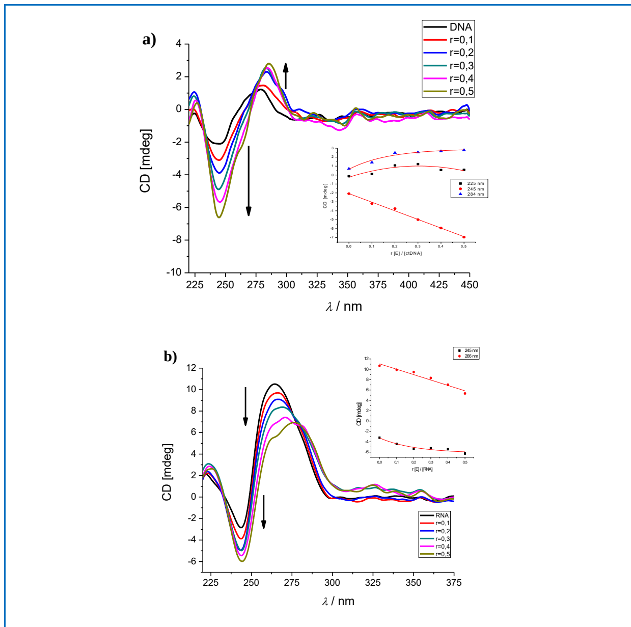
Slika 49. Promjene CD spektara otopine dl polinukleotida s dodatkom spoja E u omjeru r , u puferu natrijeva kakodilata, pri pH 7,4, I = 0,05 \text{ mol dm}^{-3} , pri 25^\circ\text{C} ; a) s ctDNA ( c_{\text{DNA}} = 2 \times 10^{-5} \text{ mol dm}^{-3} ); b) s pApU ( c_{\text{RNA}} = 2,5 \times 10^{-5} \text{ mol dm}^{-3} ); uz umetak koji se odnosi na spektralne promjene u ovisnosti o r .
