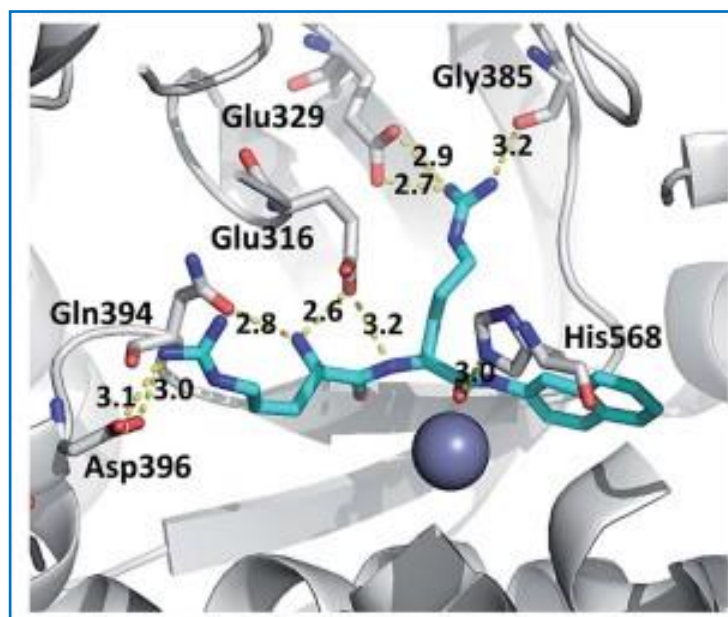
Slika 18. Prikaz vezanja komercijalnog supstrata Arg 2 -2NA (tirkizni štapići) u aktivno mjesto hDPP III (siva pozadina, gdje je Zn 2+ ion prikazan kao siva kuglica). Udaljenosti su navedene u Å. Izvor: Matovina, M. et al. New findings about human dipeptidyl peptidase III based on mutations found in cancer. RSC Adv. 7, 36326–36334 (2017).
