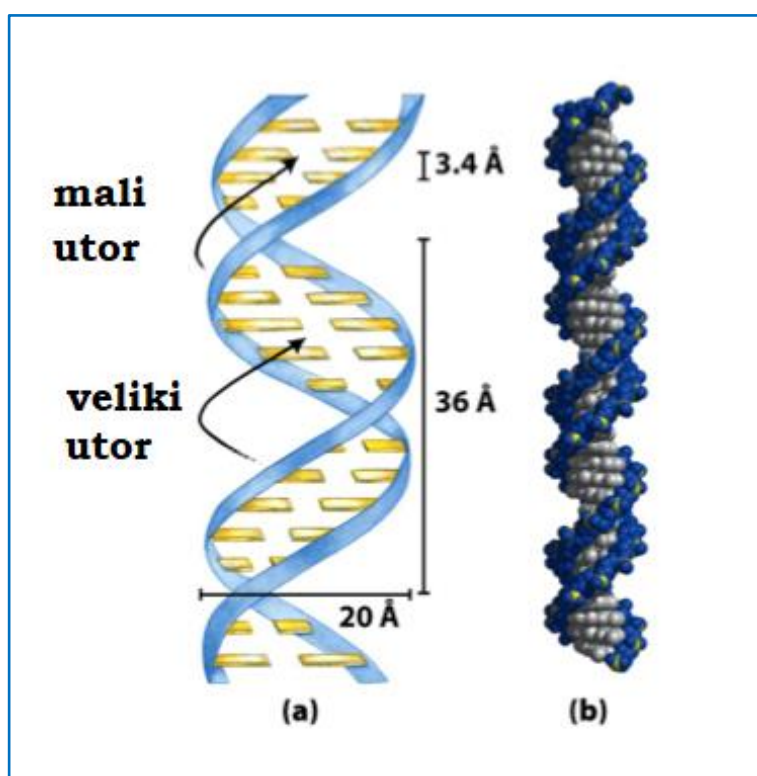
Slika 11. Prikaz strukture uzvojnice B-DNA: a) Shematski prikaz s navedenim dimenzijama uzvojnice; b) trodimenzijski prikaz (engl. space-filling model). Izvor: Prilagođeno prema Lehninger, A., Nelson, D. A. & Cox, M. M. Principles of Biochemistry . (W. H. Freeman, 2008).
