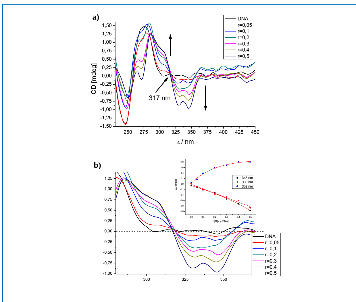
Slika 47. Promjene CD spektara otopine ctDNA ( c_{\text{DNA}} = 2 \times 10^{-5} \text{ mol dm}^{-3} ) s dodatkom spoja D r_{[C]/[DNA]} = 0,1-0,5 , u puferu natrijeva kakodilata, pri pH 7,4, I = 0,05 \text{ mol dm}^{-3} , pri 25 °C. a) CD spektar; b) uvećani dio spektra s ctDNA pod a) od 280 do 370 nm, uz umetak koji se odnosi na spektralne promjene u ovisnosti o r .
