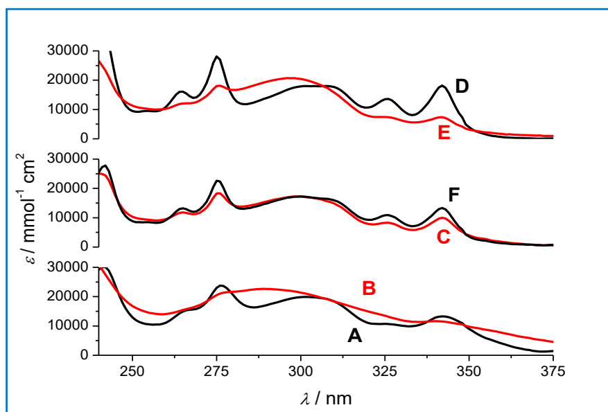
Slika 20. Usporedba UV/Vis spektara puferских otopina spojeva A-F , pH 7,0, natrijev kakodilat, I = 0,05 \text{ mol dm}^{-3} , pri 25^\circ \text{C} . Derivati s lizinskim bočnim ogrankom su prikazani crnim linijama ( A , D i F ) dok su oni s glicinskim bočnim ograncima prikazani crvenim linijama ( B , C i E ).
