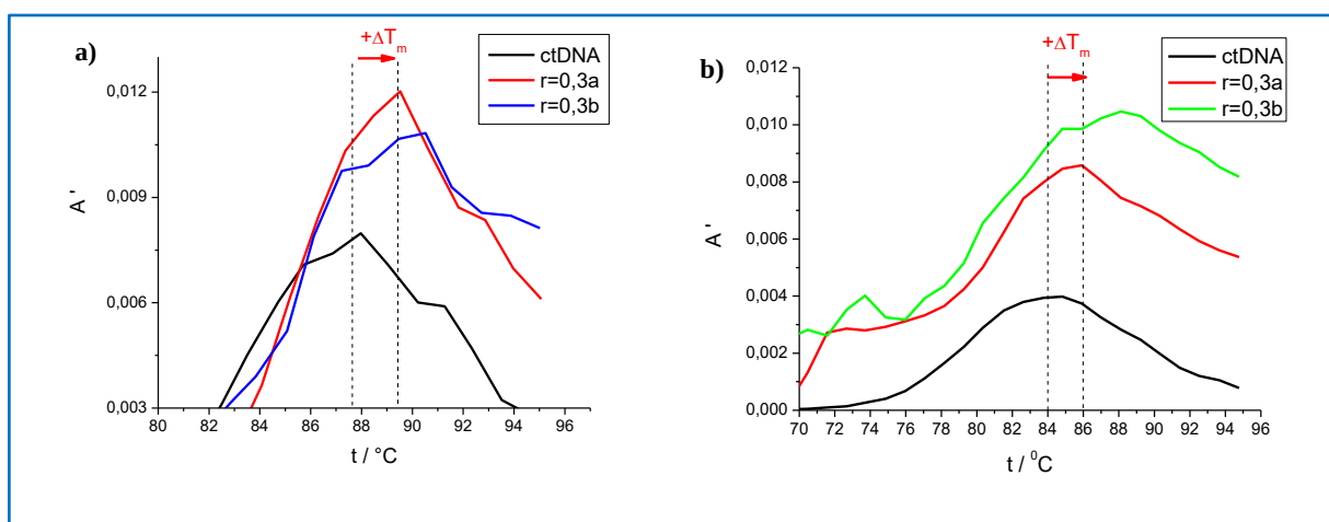
Slika 40. Prikaz krivulje temperaturne denaturacije ctDNA ( c = 2 \times 10^{-5} \text{ mol dm}^{-3} ) u prisutnosti stabilizirajućeg (pozitivan \Delta T_m pomak, crveno) spoja ( r = 0,3 ): a) A; b) E; pri pH 7,4, I = 0,05 \text{ mol dm}^{-3} .
