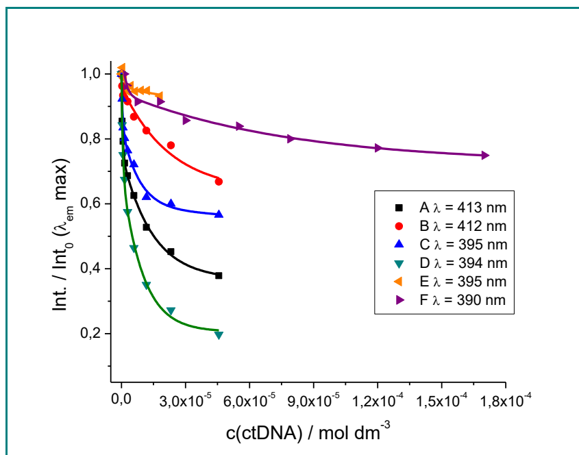
Slika 44. Usporedba rezultata fluorimetrijske titracije novოსინтетизираних спојева A-F ( c = 2 \times 10^{-7} \text{ mol dm}^{-3} , \lambda_{\text{exc}} \approx 342 \text{ nm} ) s ctDNA, u puferškoj otopini natrijeva kakodilata, pH 7,4, I = 0,05 \text{ mol dm}^{-3} pri 25^\circ \text{C} ; vrijednosti su normalizirane prema polaznom intenzitetu \text{Int}_0 pri emisiji spoja \lambda_{\text{max}} \in [390-415] \text{ nm} .
