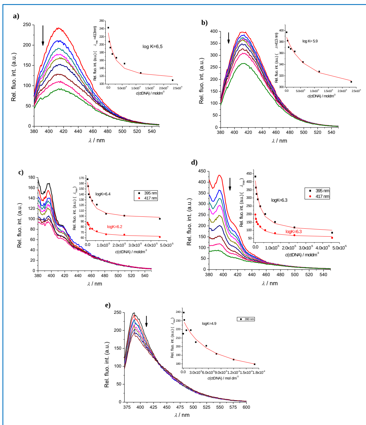
Slika 42. Promjene fluorescencijskih spektara puferskih otopina novოსინтетизираних спојева: a) A ; b) B ; c) C ; d) D ; e) F ; ( c = 2 \times 10^{-7} \text{ mol dm}^{-3} ; pH 7,4; I = 0,05 \text{ mol dm}^{-3} ) pri različitim koncentracijama dodanih alikvota stock otopine ctDNA ( c_0 = 5,3 \times 10^{-3} \text{ mol dm}^{-3} ) pri 25 °C, \lambda_{\text{exc}} = 342 \text{ nm} , inkubacijsko vrijeme 10 sekundi.
