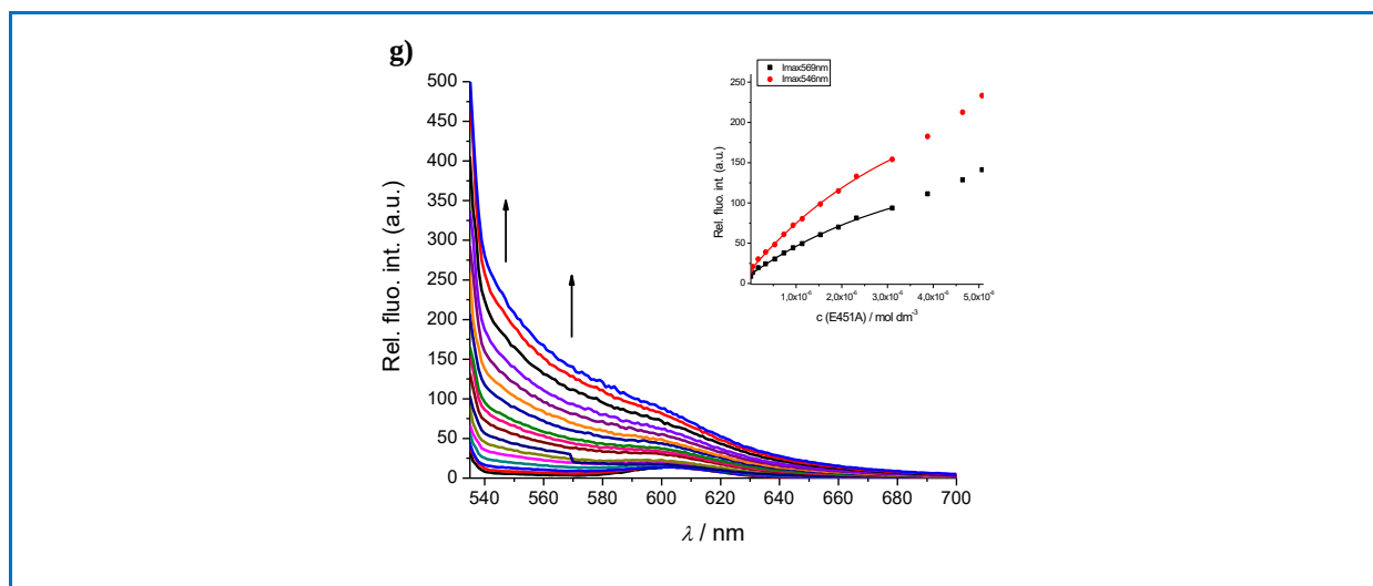
Slika 24. Promjena fluorescencijskog spektra puferskih otopina novosintetiziranog spoja: g) CIA ; ( c = 1 \times 10^{-8} \text{ mol dm}^{-3} ; pH 7,4; I = 0,05 \text{ mol dm}^{-3} ) pri različitim koncentracijama dodanih alikvota ishodišne otopine inaktivnog E451A ( c_0 = 1,8 \times 10^{-4} \text{ mol dm}^{-3} ; koncentracijski raspon od \approx 1 \times 10^{-7} \text{ mol dm}^{-3} - 4,4 \times 10^{-6} \text{ mol dm}^{-3} ) pri 25 °C.
