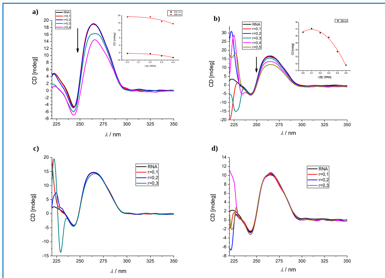
D-Slika 16. Promjene CD spektara otopine pApU ( c_{\text{RNA}} = 2,5 \times 10^{-5} \text{ mol dm}^{-3} ), u puferu natrijeva kakodilata, pri pH 7,4, I = 0,05 \text{ mol dm}^{-3} , pri 25^\circ \text{C} , \lambda_{\text{exc}} = 342 \text{ nm} , slitovi 10 – 10, inkubacijsko vrijeme 0 sekundi, s dodatkom novosintetiziranog spoja: a) A ; b) B ; c) C ; d) F ; u navedenom pripadnom stehiometrijskom omjeru r .
