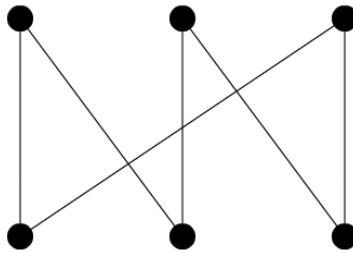
Slika 2.5: Pojednostavnjenje incidencijske strukture
