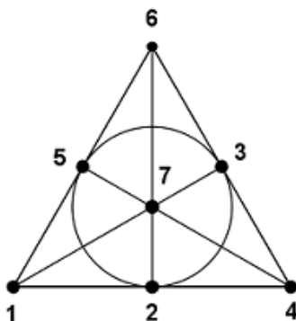
Slika 1.3: Simetrični 2-(7, 3, 1) dizajn
