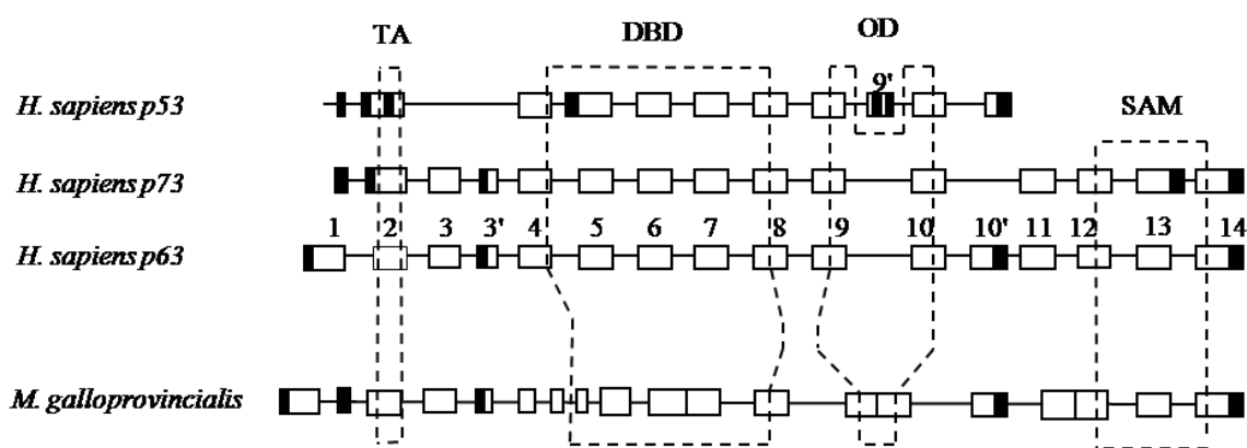
Slika 18. Shema sravnjenja gena porodice p53 čovjeka (p53, p63 i p73) i gena porodice p53 M.galloprovincialis . Egzoni su prikazani pravokutnicima (crno su označeni UTR-ovi), a introni ravnim linijama. Očuvane domene porodice p53 (TA, DBD, OD i SAM) uokvirene su iscrtkanim linijama.
