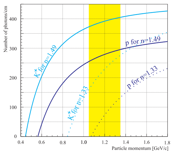
SLIKA 2.13: OVISNOST BROJA PRODUCIRANIH FOTOELEKTRONA U ČERENKOVLEJIM DETEKTORIMA O IMPULSU KAONA I PROTONA ZA DVA RAZLIČITA RADIJATORA: VODA ( n=1.33 ) I AKRILNI RADIJATOR ( n=1.49 ). OBOJANO PODRUČJE REPREZENTIRA IMPULSNU AKCEPTANCIJU HKS-A.
