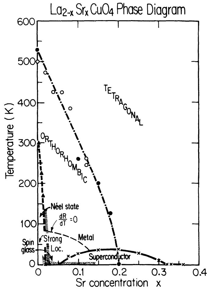
Slika 5.5: Fazni dijagram \text{La}_{2-x}\text{Sr}_x\text{CuO}_4 . Slika je preuzeta iz [51].
