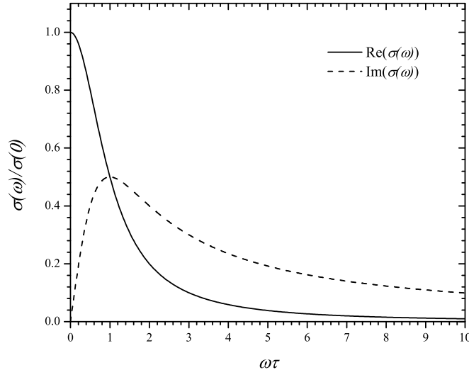
Slika 2.1: Realan (puna linija) i imaginaran (crtkana linija) dio vodljivosti Drudeova modela u slučaju periodične pobude.
