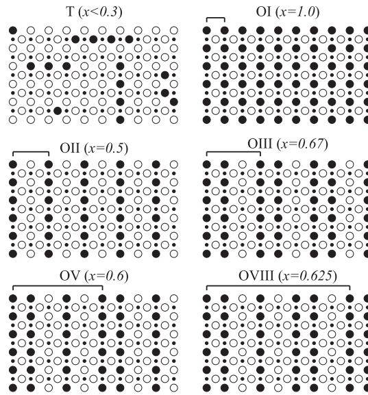
Slika 5.3: Periodični uzorci i imena pripadnih faza Cu–O lanaca u YBCO kristalu. T označava nasumičan razmještaj kisika (tetragonalna simetrija), a O različite ortorompske faze Cu–O lanaca s tipičnim dopiranjem za pojedinu fazu. \circ su prazne, a \bullet popunjene pozicije kisika.
