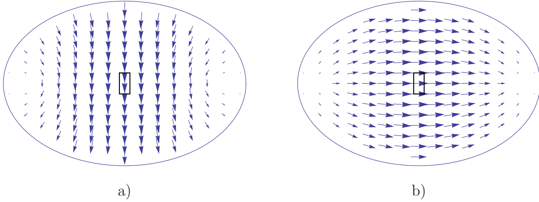
Slika 4.9: Dvdimenzionalna raspodjela polja u ravнини uzorka (naznačen crnim pravokutnikom) za modove {}^eTE_{111} i {}^eTE_{112} . Obratite pozornost da se u slučaju a) radi o raspodjeli električnog polja, a b) magnetskog polja.
