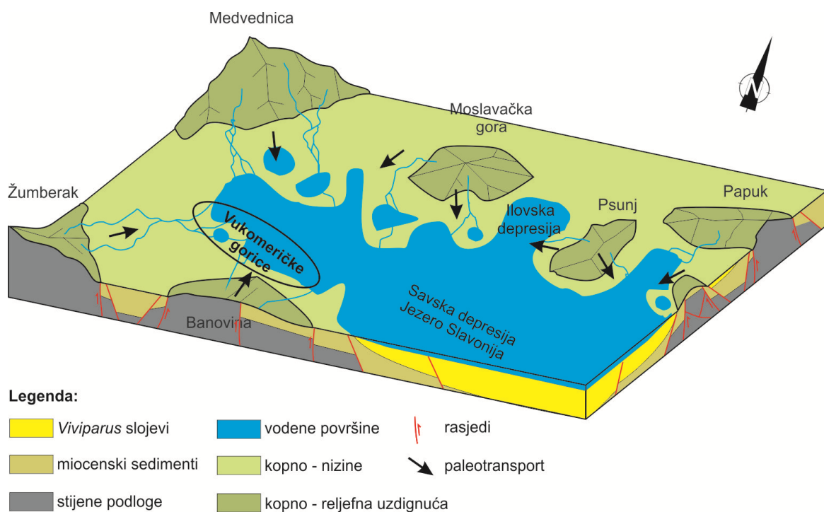
Slika 5.23. Rasprostriranje jezerskih okoliša u Savskoj depresiji tokom perioda taloženja gornjih Viviparus slojeva. Položaj današnjih Vukomeričkih gorica označen je elipsom.
