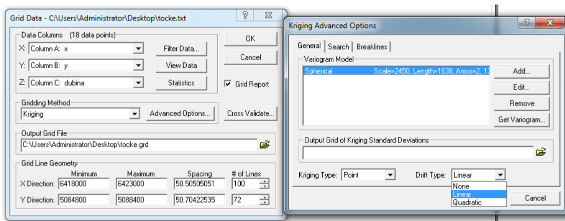
Slika 6.6. Primjer sučelja u Surferu
