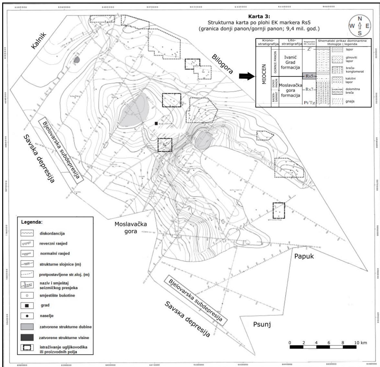
Slika 4.6. Strukturalna karta Bjelovarske subdepresije po plohi EK markera Rs5 (Malvić, 2011)
