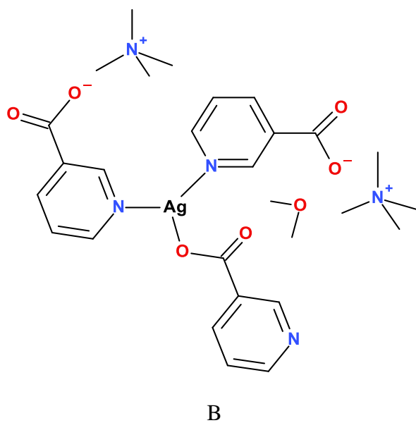
Slika 18. Koordinacijsko okruženje oko iona srebra(I) kod spojeva A) catena-[[piridin-3-karboksilato-(O,O')]srebra(I)] i B) amonijeva bis[piridin-3-karboksilato-(O,N,N')] argentata(I) monohidrata.
