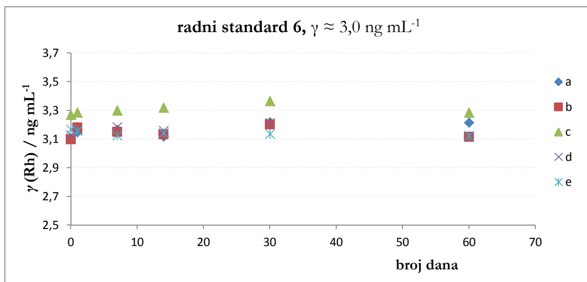
Slika J1c. Stabilnost radnih standarda rodija, a) 5 % HNO 3 (v/v), b) 5 % HNO 3 / 1 % HCl (v/v), c) 5 % HNO 3 / 2 % HCl (v/v), d) 5 % HNO 3 / 5 % HCl (v/v) i e) 1 % HCl (v/v)
