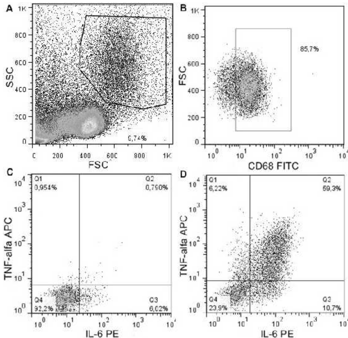
Slika 11. Primjer postavljanja elektronskih ograda za mjerenje proizvodnje citokina od strane monocita. A) Elektronska ograda postavljena oko populacije monocita definiranih na temelju veličine (FSC) i zrnatosti (SSC) stanica; B) monociti su dalje preciznije ograničeni na temelju izraženosti biljega CD68; C) na dvoparametarskom dijagramu fluorescencije IL-6 i TNF- \alpha identificirani su nestimulirani monociti a D) monociti stimulirani LPS-om koji
