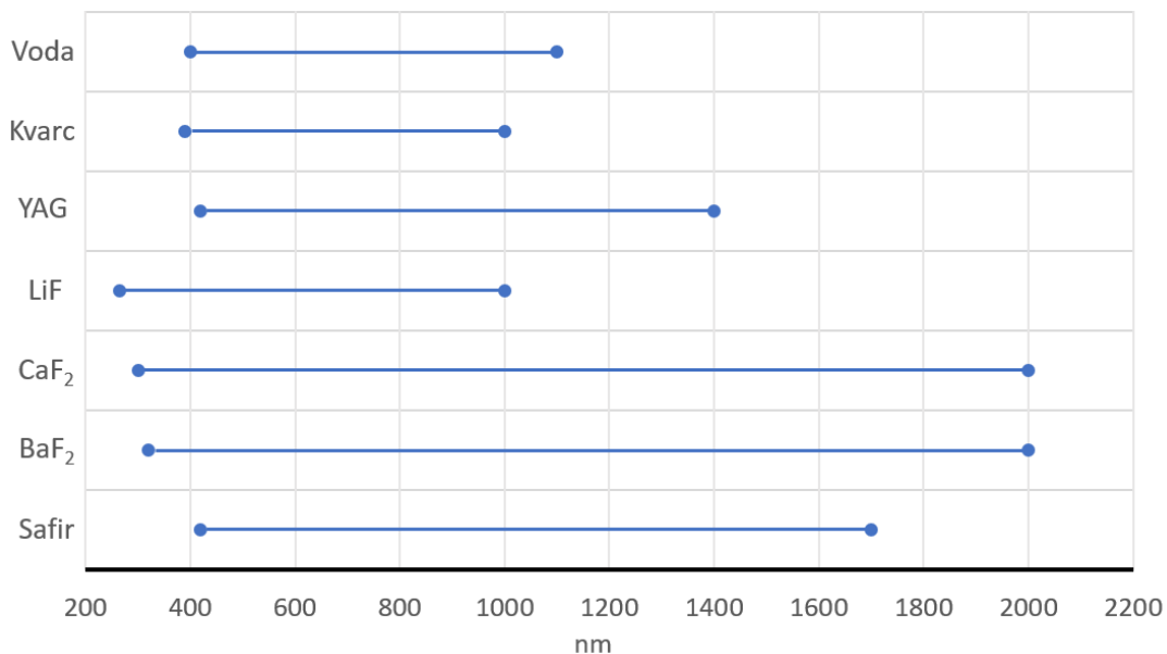
Slika 1.4: Pregled eksperimentalno mjerenih superkontinuumu stvorenih pumpnom valnom duljinom od 800nm u raznim materijalima. Podaci su preuzeti iz: voda - [43], kvarc - [44], YAG, safir - [45], \text{BaF}_2 , \text{CaF}_2 - [46], LiF - [47].
