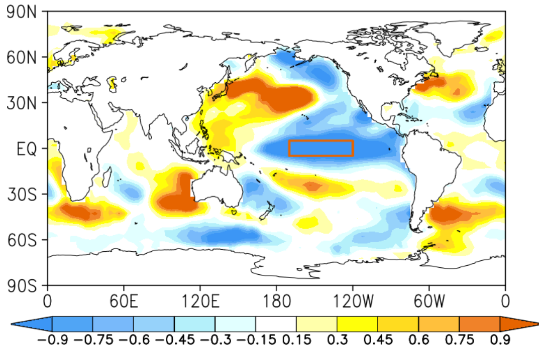
(b) Niño3.4 region
