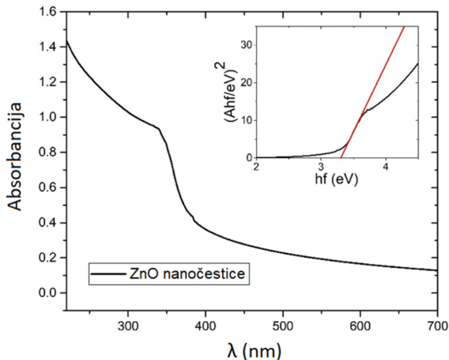
Slika 50: Fotoapsorpcijski spektar ZnO koloidne otopine; Umetak: Taucov graf za računanje indirektna širine zabranjenog pojasa
