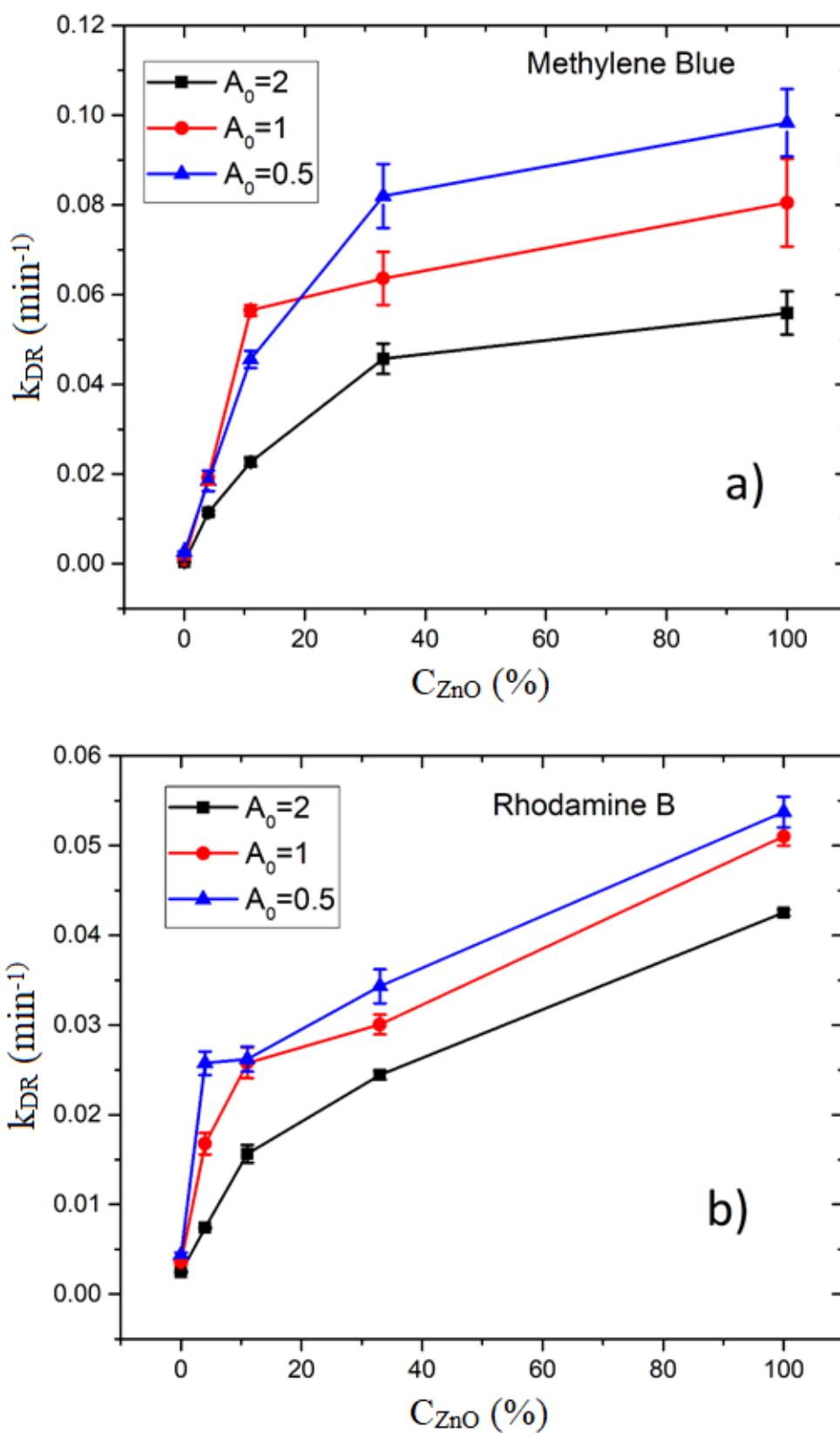
Slika 54: Fotodegradacijske konstante ( k_{DR} ) za raspad a) MB i b) RB u ovisnosti o koncentraciji ZnO katalizatora za različite početne koncentracije bojila
