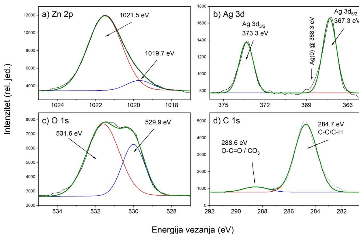
Slika 58: Visokorezolucijski spektri ZnO nanočestica dopiranih srebrom (3000 pulseva korišteno za depoziciju srebra u PLD) i prilagodbe za a) Zn 2p 3/2 , b) Ag 3d, c) O 1s i d) C 1s
