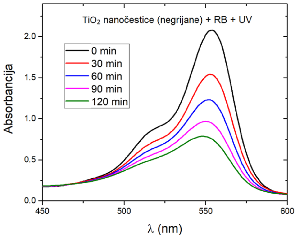
Slika 35: Fotodegradacija Methylene Blue u prisutnosti negrijanih \text{TiO}_2 nanočestica tijekom ozračivanja UV zračenjem
