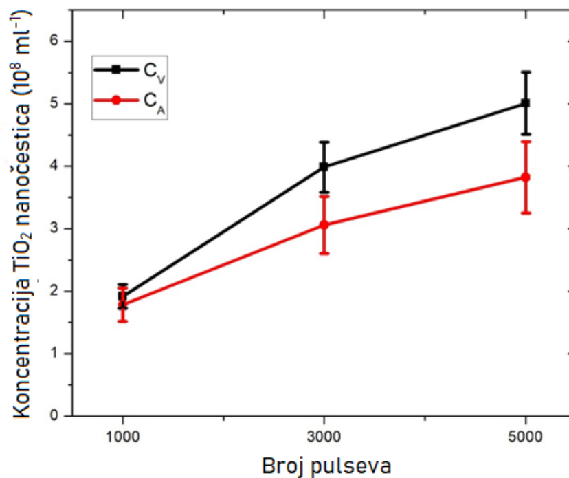
Slika 20: Ovisnost koncentracije \text{TiO}_2 nanočestica u koloidnim otopinama o broju pulseva, za dva različita načina računanja koncentracije: preko volumena kratera ( C_V ) i preko absorpcije ( C_A )
