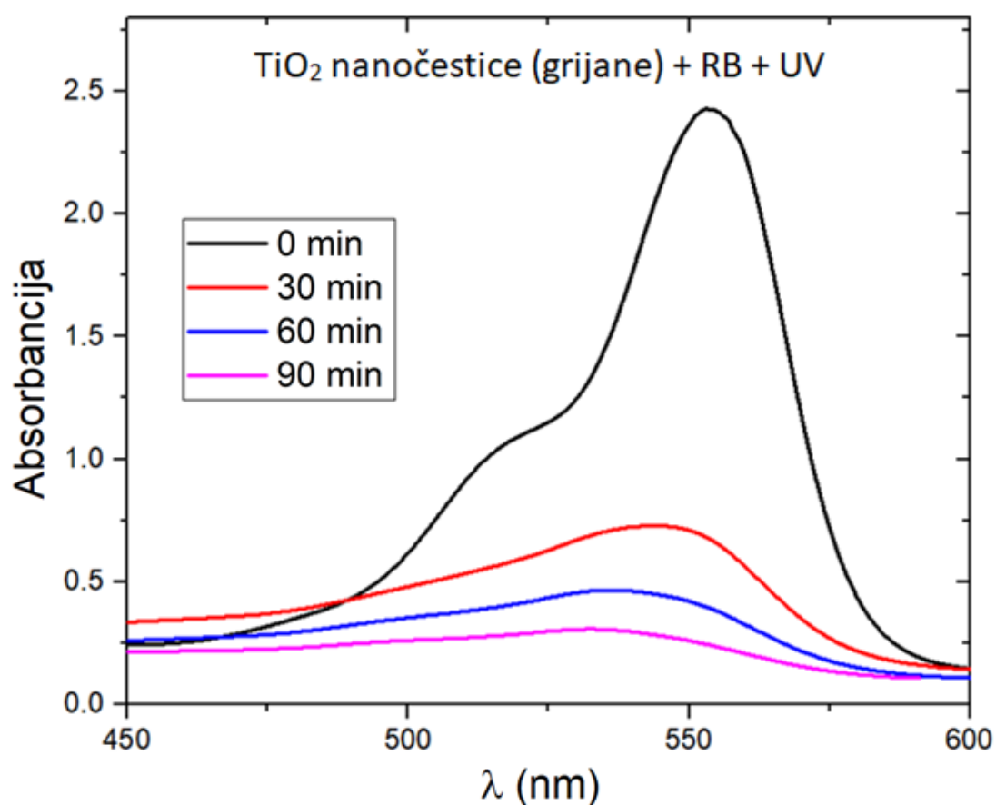
Slika 36: Fotodegradacija Rhodamine B u prisutnosti grijanih \text{TiO}_2 nanočestica tijekom ozračivanja UV zračenjem
