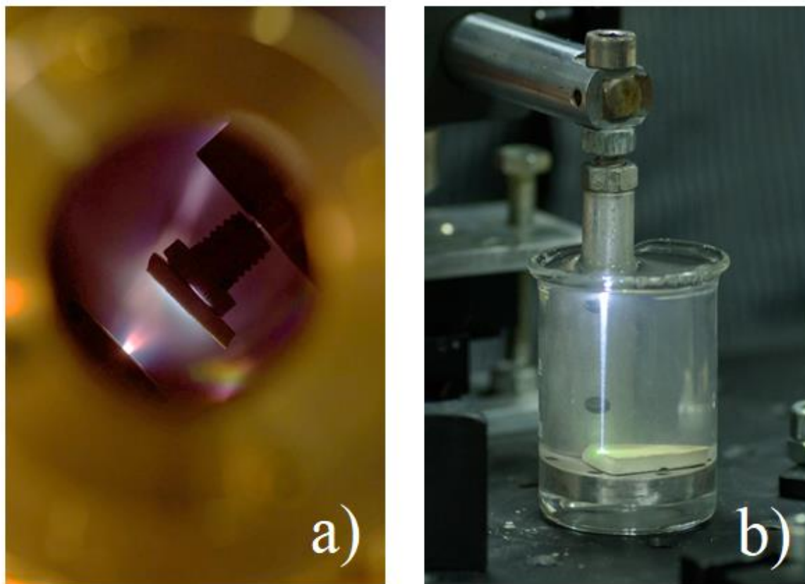
Slika 11: a) Naparavanje ZnO supstrata srebrom u PLD komori; b) Laserska ablacija ZnO mete prekrivene filmom srebra za sinteza ZnO nanočestica dopiranih srebrom
