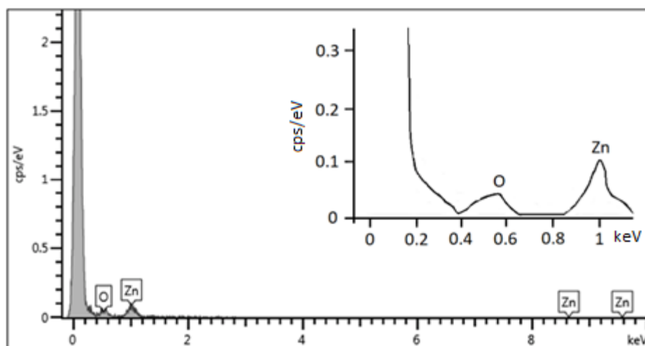
Slika 45: EDS mjerenje na ZnO nanočestici (umetak: uvećan prikaz glavnih vrhova za O i Zn)
