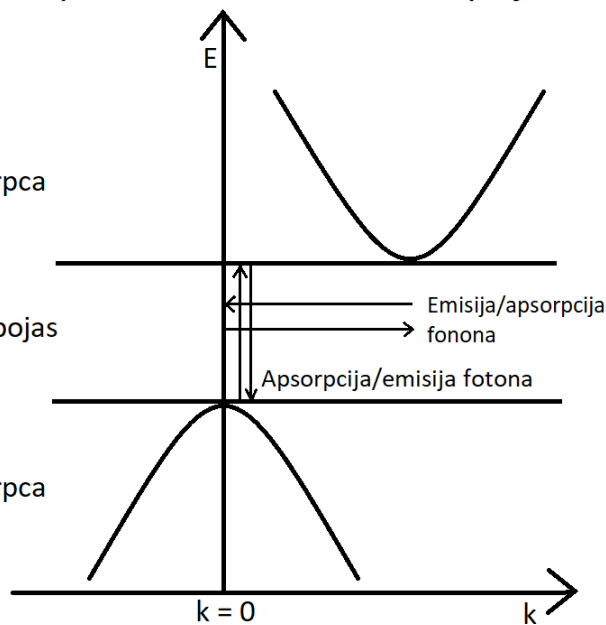
Slika 2: Sheme energijskog dijagrama za elektronske prijelaze u slučaju a) direktnog i b) indirektnog zabranjenog pojasa
