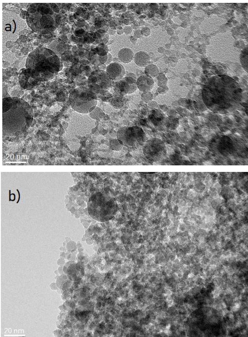
Slika 24: Primjeri TEM snimki \text{TiO}_2 nanočestica (a – negrijane, b – grijane)
