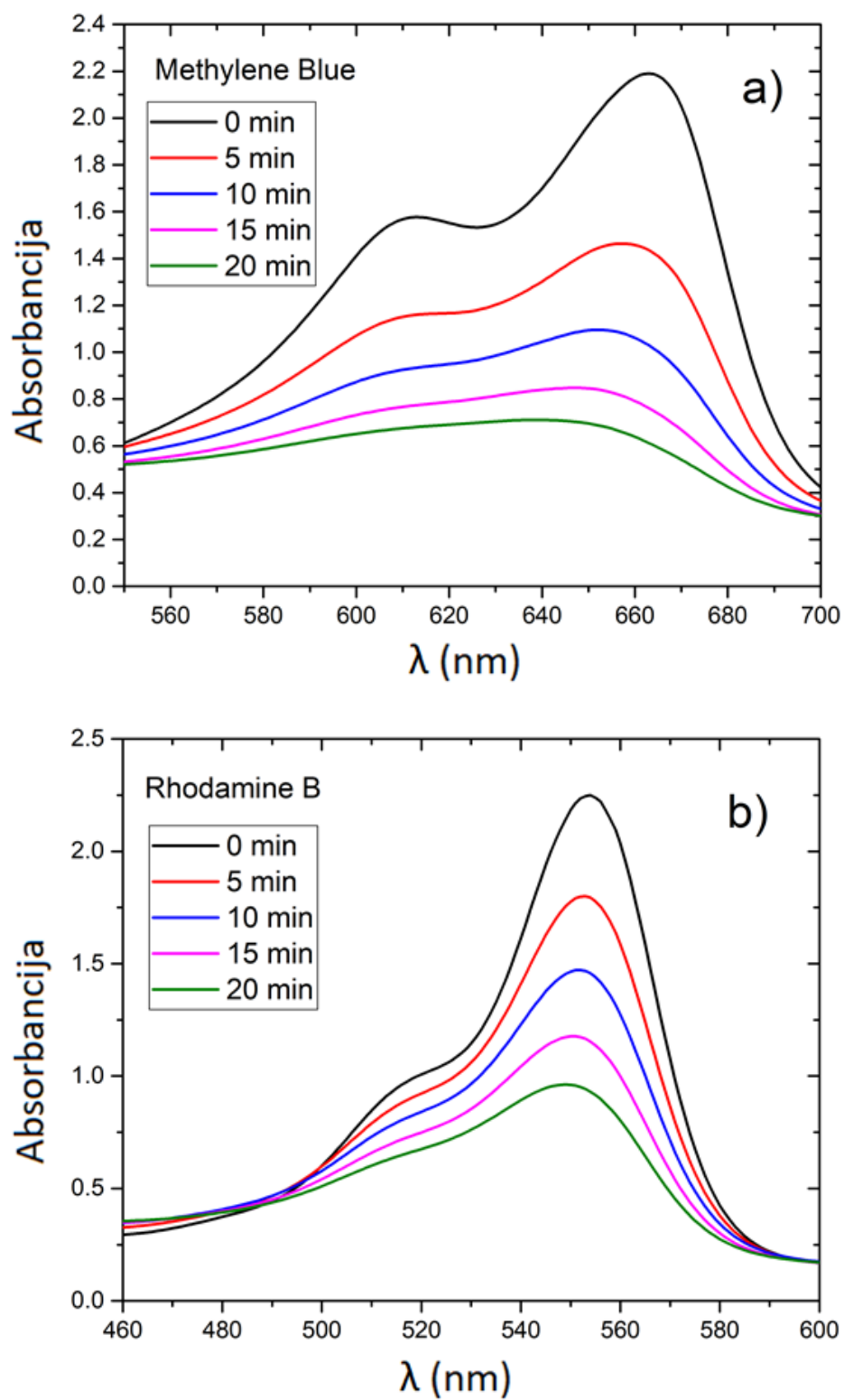
Slika 51: Fotodegradacija a) MB i b) RB u nerazrijeđenoj koloidnoj otopini ZnO ( C_{\text{ZnO}} = 100\% ) tijekom ozračivanja UV zračenjem
