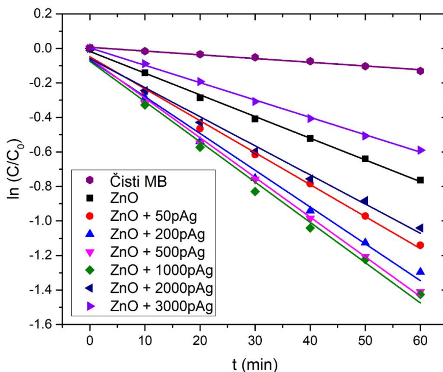
Slika 64: \ln(C/C_0) u ovisnosti o vremenu za fotokatalitičku degradaciju MB u različitim koloidnim otopinama ZnO nanočestica dopiranih srebrom pod UV zračenjem
