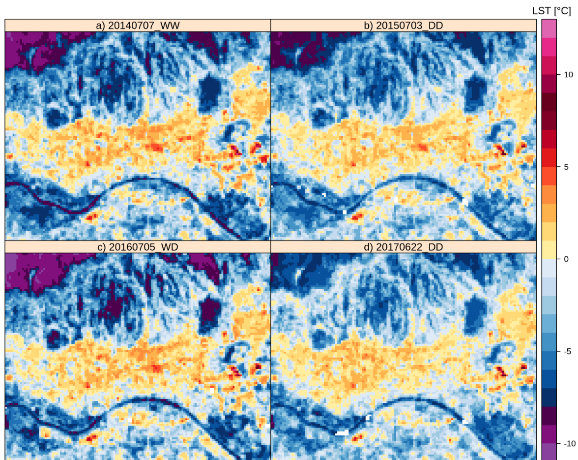
Slika 5.3.8 Razlika u površinskoj temperaturi tla (LST) i prosječnoj vrijednosti LST-a za najgušće izgrađene klase (LU1, LU2 i LU7) za odabrani ljetni dan koji odgovara situaciji: a) vlažno-vlažno (20140707_WW), b) sušno-sušno (20150703_DD), c) vlažno-sušno (20160705_WD) i d) sušno-sušno (20170622_DD).
