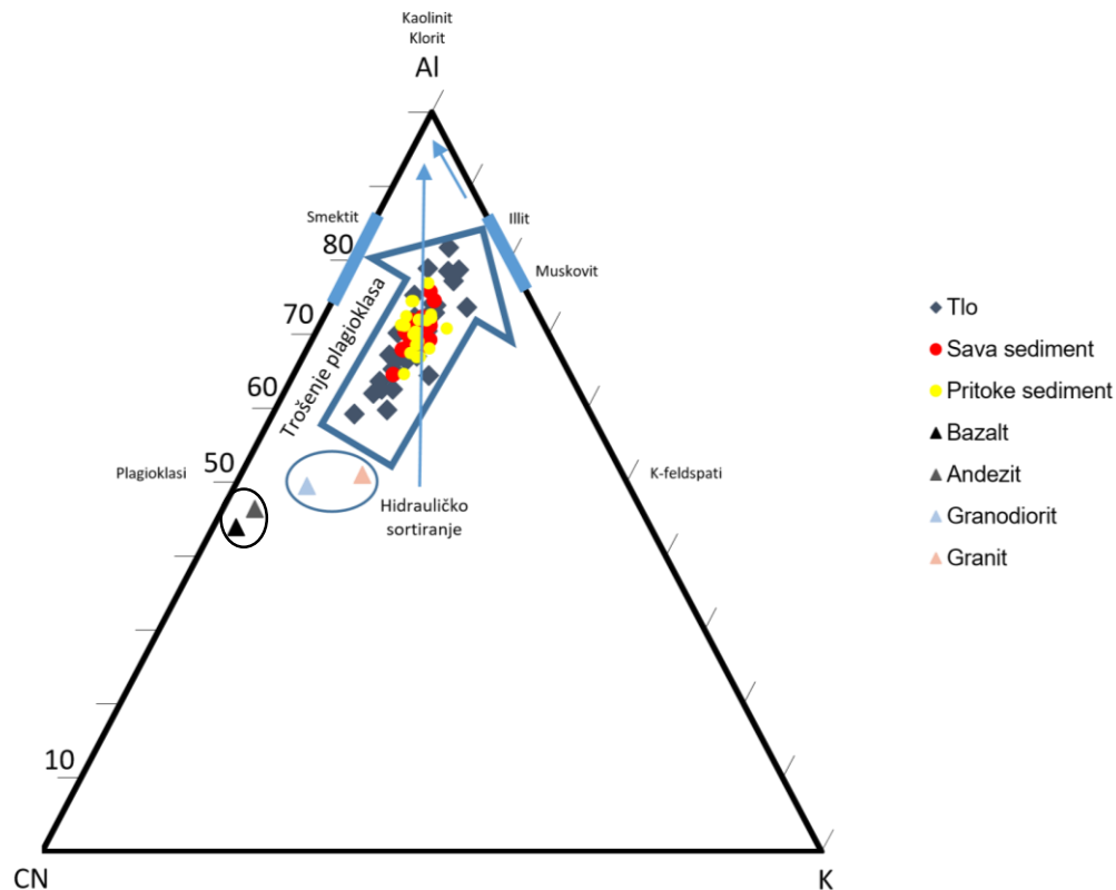
Slika 64. A-CN-K ternarni dijagram s navedenim CIA indeksom kemijskog trošenja za istraživane uzorke i potencijalno izvorišne stijene (Taylor i McLennan, 1985)
