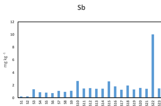
Slika 40. Raspodjela Li, Mn, Mo, Nb, Ni, Pb, Rb i Sb u sedimentima duž gornjeg toka rijeke Save
