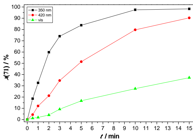
Slika 62. Nastajanje fotoproducta 71 tijekom ozračivanja spoja 14 u CH 3 OH-H 2 O (4:1) zračenjem različitih valnih duljina.
