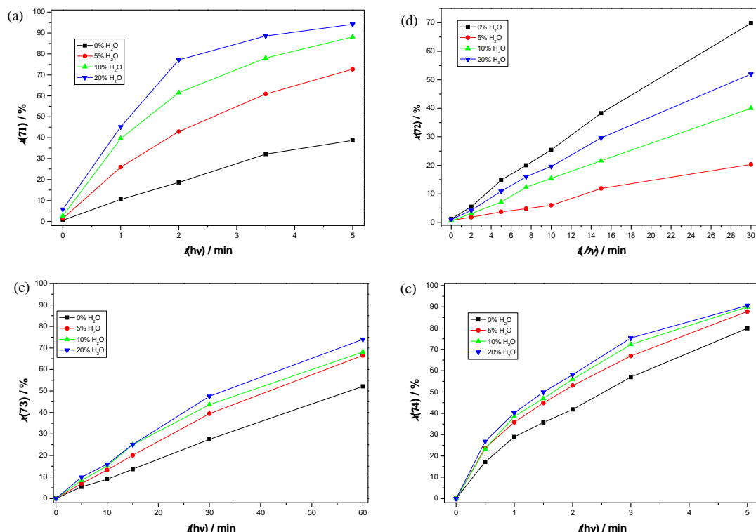
Slika 63. Ovisnost udjela fotoprodukta o udjelu vode u metanolu i o vremenu ozračivanja za spoj: (a) 14 ; (b) 15 ; (c) 16 i (d) 17 .
