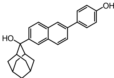
Prilog 36. ^1\text{H} NMR (300 MHz, DMSO- d_6 ) i ^{13}\text{C} NMR (150 MHz, DMSO- d_6 ) spektri ( \delta/\text{ppm} ) 6-(2-hidroksi-2-adamantil)-2-(4-hidroksifenil)naftalena ( 12 ).
