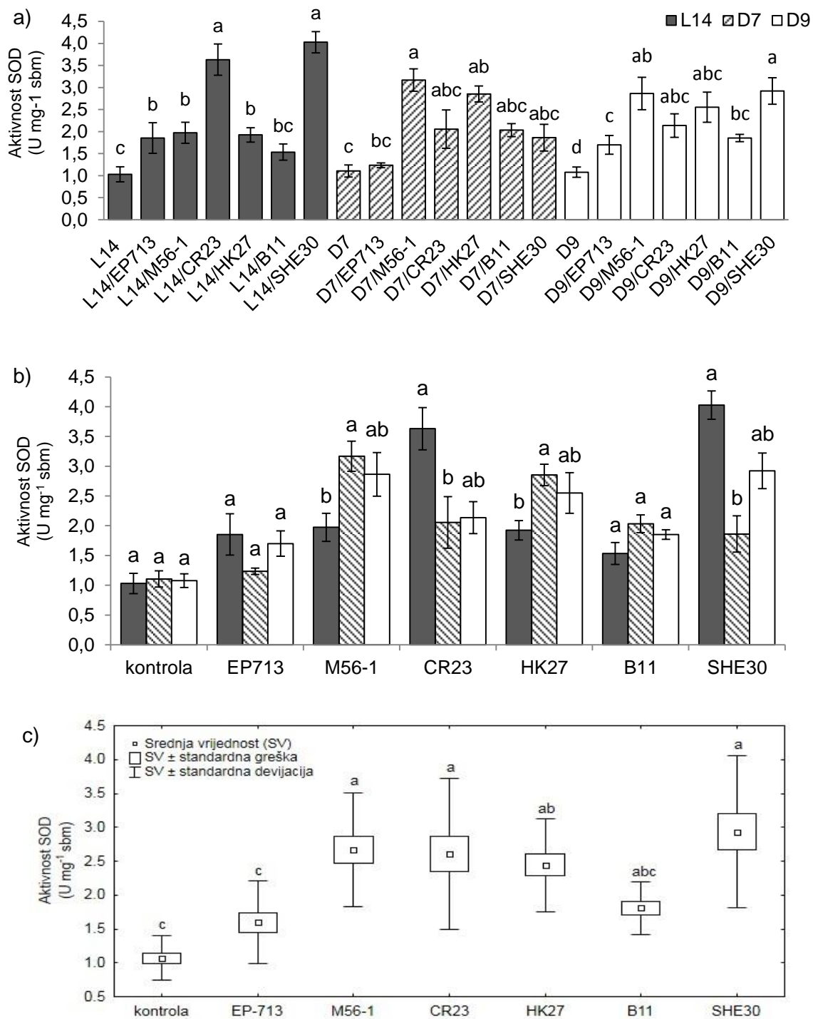
Slika 20. Utjecaj različitih sojeva virusa CHV1 na aktivnost superoksid dismutaze (SOD) gljive Cryphonectria parasitica ; a) Utjecaj raznih virusnih sojeva na isti izolat gljive; b) Utjecaj pojedinačnih virusnih sojeva na različite izolate gljive; c) Objedinjeni utjecaj svakog pojedinačnog virusnog soja na rast svih triju izolata gljive. Oznake na grafičkim prikazima iste su kao na Slici 15. Sve statističke procjene provedene su na razini značajnosti p < 0,05 .
