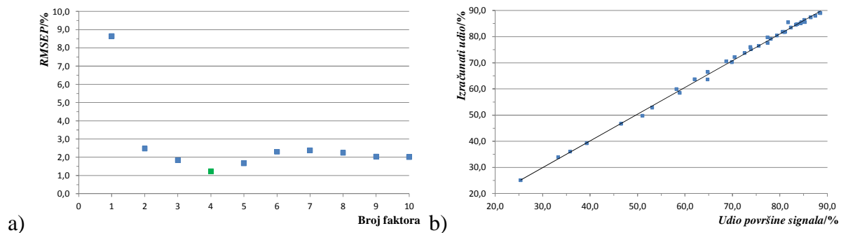
a) Ovisnost vrijednosti RMSEP o broju faktora i b) regresijski pravac validacije modela 1-B-2 za spoj 2 s 4 faktora.
