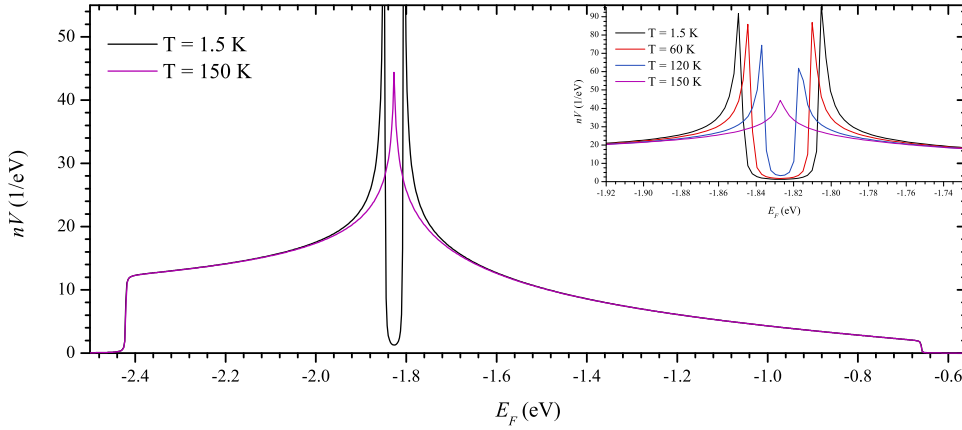
Slika 2.6: Otvaranje procjeka u gustoći stanja na različitim temperaturama T \leq T_{CDW} u ovisnosti o E_F .
