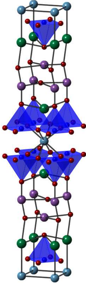
Slika 5.6: Kristalna struktura spoja Bi 2 Sr 2 CaCu 2 O 8+δ .
