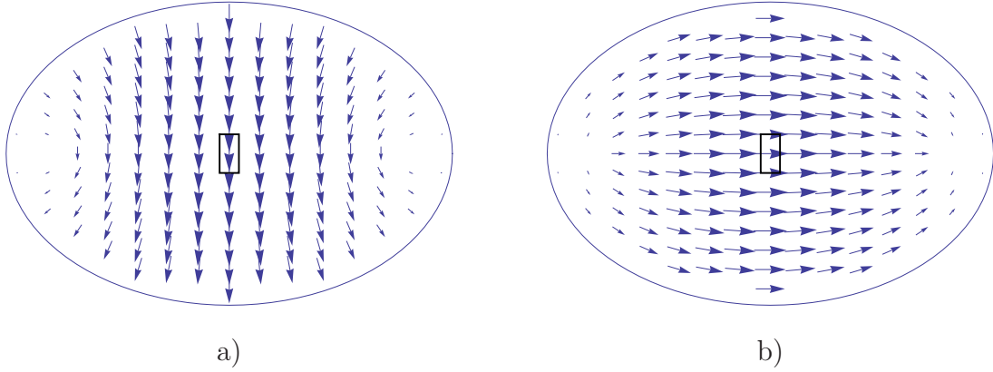
Slika 4.9: Dvodimenzionalna raspodjela polja u ravнини uzorka (naznačen crnim pravokutnikom) za modove {}^eTE_{111} i {}^eTE_{112} . Obratite pozornost da se u slučaju a) radi o raspodjeli električnog polja, a b) magnetskog polja.
