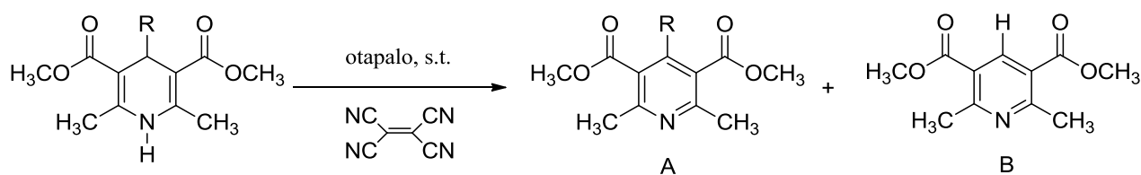
Tablica 55. Dealkilacija 2,6-dimetil-3,5-di(metoksikarbonil)-4-alkil-1,4-DHP s TCNE na sobnoj temperaturi
