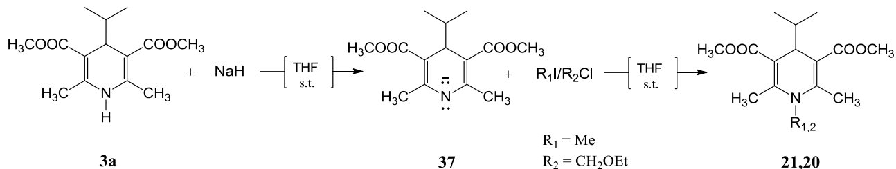
Tablica 29: Sinteza N-derivata 2,6-dimetil-3,5-di(metoksikarbonil)-4-izopropil-1,4-DHP prema Shemi 28
