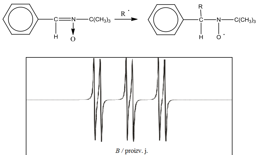
Slika 33: EPR spektar PBN – radikal adukta
