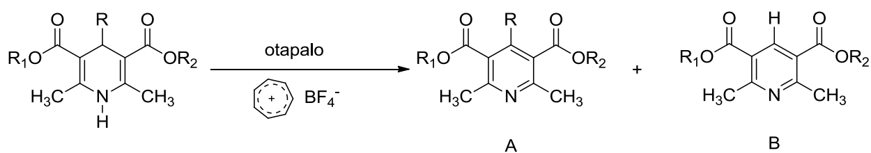
Tablica 52. Dealkilacija 2,6-dimetil-3,5-di(alkiloksikarbonil)-4-alkil-1,4-DHP s tropilijevim tetrafluoroboratom
