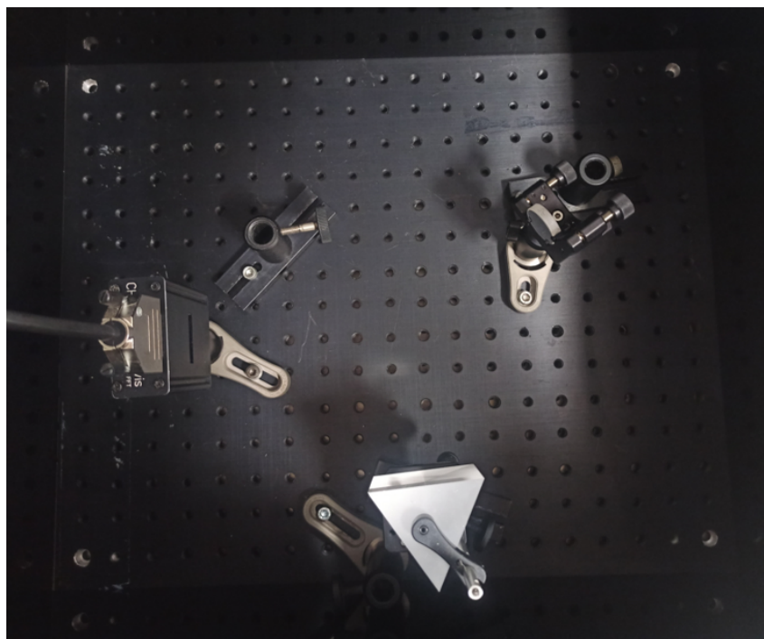
Slika 3.6: Sustav za detekciju kućne izrade.
