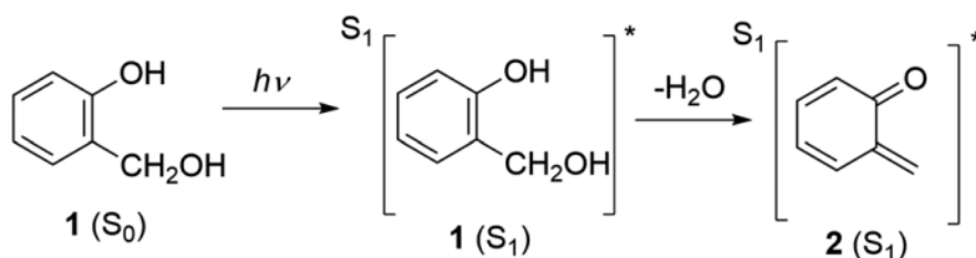
Slika 6.1: Fotodehidratacija o -hidroksimetilfenola ( 1 ) i dobivanje QM u pobuđenom stanju ( 2 ).
