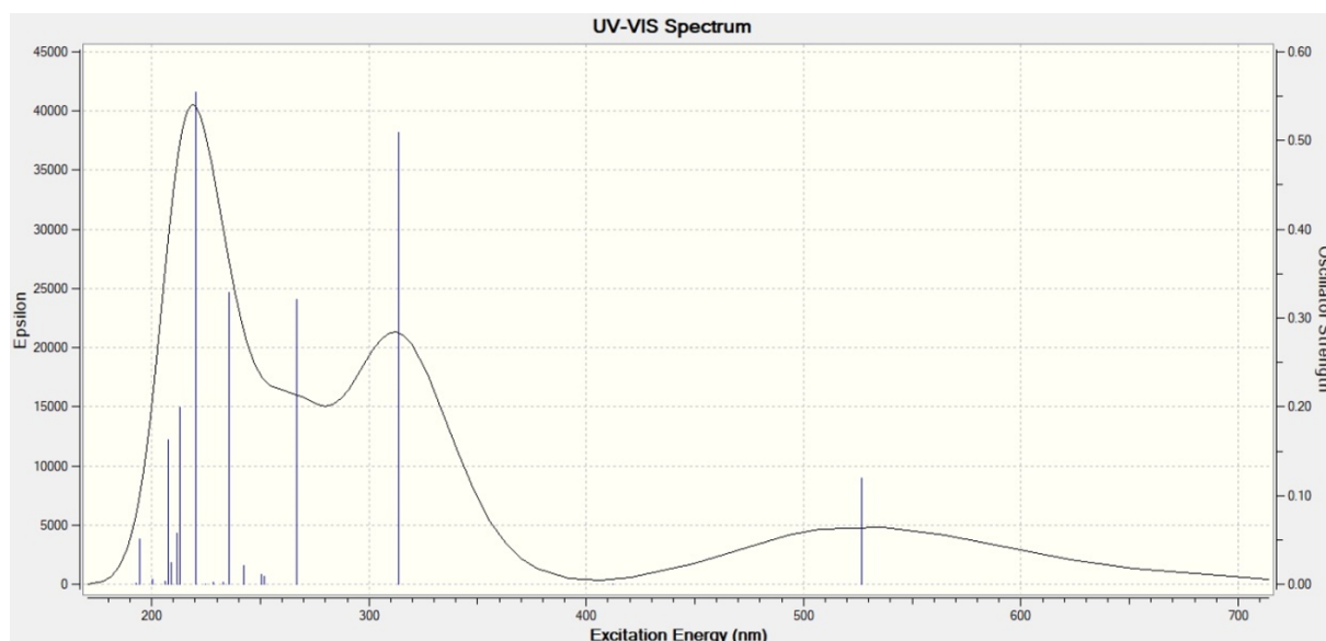
Slika 7.21: Rezultat računskih simulacija apsorpcijskog spektra stanja 2-QM ( S_0 ).
