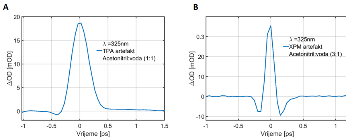
Slika 1.13: Vremenski profili artefakata TA metode u čistom otapalu na valnoj duljini od 325nm. A) TPA artefakt dobiven u mješavini acetonitrila i vode (1:1) na snazi pumpnog pulsa od 1.2mW. B) XPM artefakt dobiven u mješavini acetonitrila i vode (3:1) na snazi pumpnog pulsa od 0.22mW.
