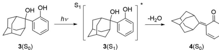
Slika 6.2: Fotokemijsko stvaranje QM-a 4(S 0 ).
