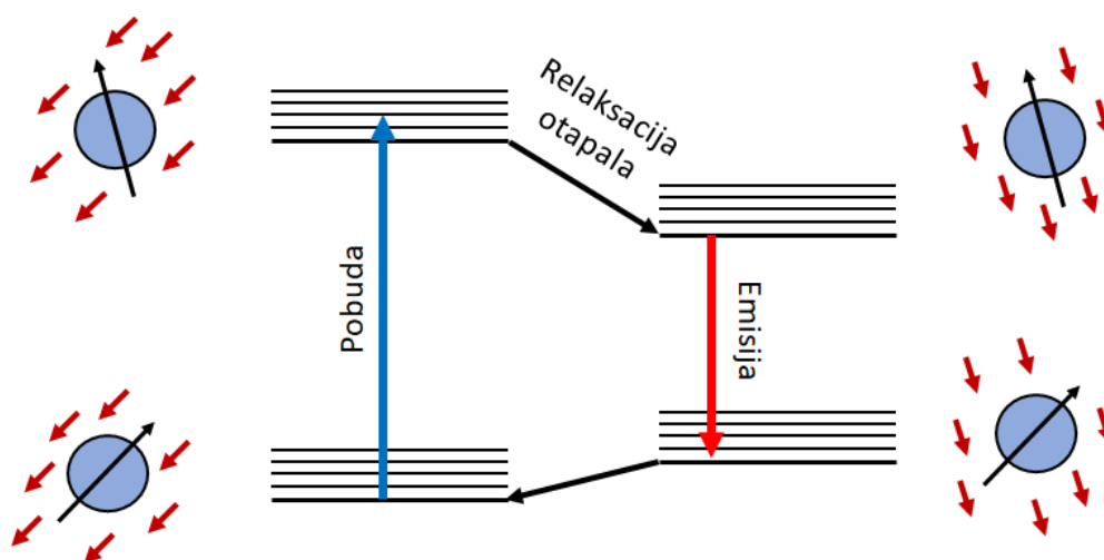
Slika 2.6: Tijekom reorijentacije polarnog otapala oko molekule DCM dolazi do snižavanja energije pobuđenog stanja što kao posljedicu ima kontinuiranu promjenu valnih duljina stimulirane emisije i apsorpcije višeg stanja. Crvenim strelicama označeni su dipolni momenti molekula polarnog otapala dok su crnim strelicama označeni dipolni momenti DCM-a.
