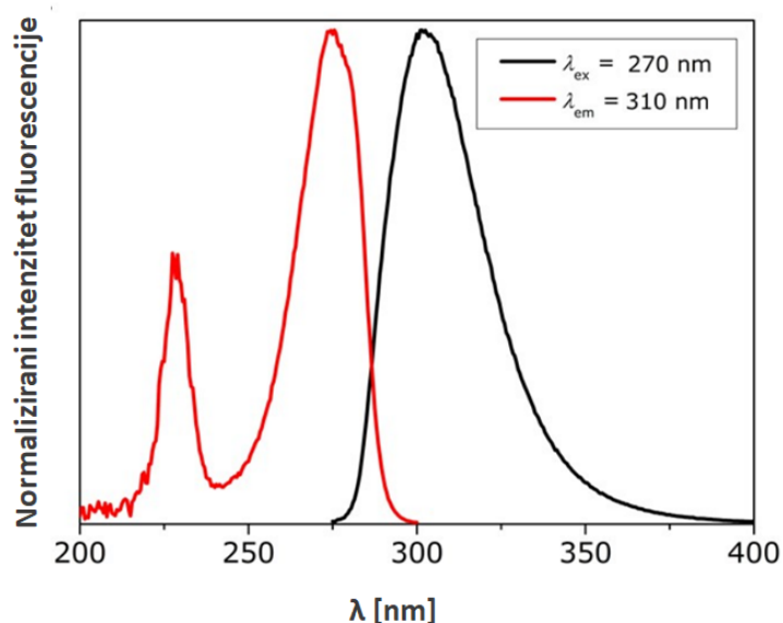
Slika 6.3: Normalizirani ekscitacijski (crveno) i emisijski (crno) spektri molekule 3 u \text{CH}_3\text{CN-H}_2\text{O} (1:1). Naznačene su emisijska i ekscitacijska valna duljina.
