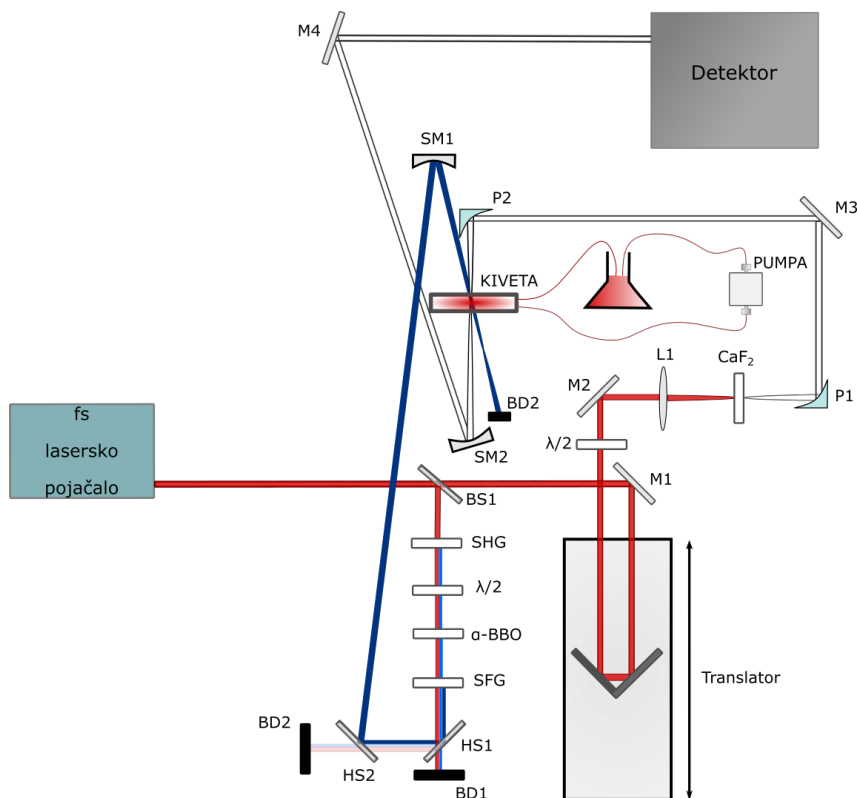
Slika 3.2: Postav za ultrabrznu tranzijentnu apsorpciju korišten u eksperimentu. Oznake: BS - djeliteљи snopa, L - leće, M - zrcala, S - prekidači zrake, HS - separatori harmonika
