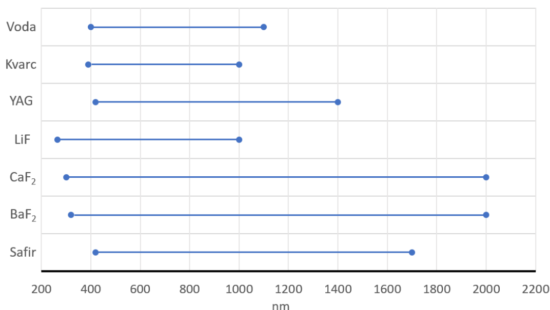
Slika 1.4: Pregled eksperimentalno mjerenih superkontinuum stvorenih pumpnom valnom duljinom od 800nm u raznim materijalima. Podaci su preuzeti iz: voda - [43], kvarc - [44], YAG, safir - [45], \text{BaF}_2 , \text{CaF}_2 - [46], LiF - [47].
