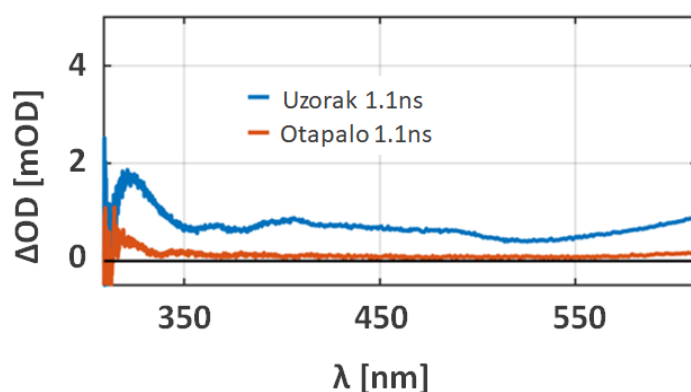
Slika 7.8: Usporedba TA spektara uzorka 1 (plavo) i otapala (narančasto) u zadnjoj dostupnoj vremenskoj točki (1.1ns). Povećana apsorpcija uzorka na duljim valnim duljinama (>500nm) ukazuje na povećanu koncentraciju otopljenih elektrona u otopini uzorka što ukazuje na stvaranje radikal kationa.
