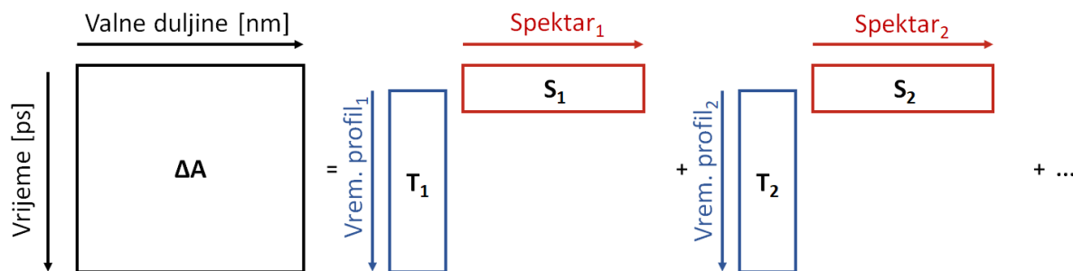
Slika 2.4: Shematski prikaz globalne analize eksperimentalnih podataka dobivenih određenom metodom ultrabrze spektroskopije. Matrica \Delta A se dekomponira na vremenske profile T_i te pridružene spektre S_i .
