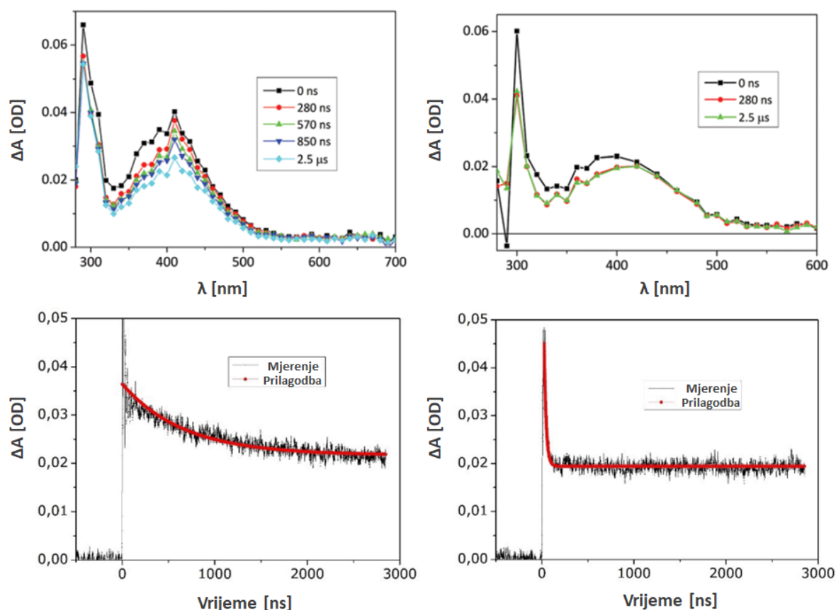
Slika 6.8: ns-TA (LFP) mjerenja molekule 3 otopljene u \text{CH}_3\text{CN-H}_2\text{O} (1:1) koncentracije c = 2.0 \times 10^{-4} \text{ M} . Prikazani su spektri u vremenu i prilagodba mono-eksponencijalne funkcije na kinetički profil na 400nm. Lijevo - mjerenja uzorka propuhanog mlazom argona i desno - uzorak propuhan mlazom \text{O}_2 . Energija laserskog pulsa valne duljine 266nm podešena je na 17mJ po pulsu.
