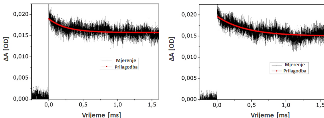
Slika 6.9: ms-TA (LFP) mjerenja molekule 3 otopljene u \text{CH}_3\text{CN-H}_2\text{O} (1:1) koncentracije c = 2,0 \times 10^{-4} \text{ M} . Prikazana je prilagodba mono-eksponencijalne funkcije na kinetički profil na 400nm. Lijevo - mjerenja uzorka propuhanog mlazom argona i desno - uzorak propuhan mlazom \text{O}_2 . Energija laserskog pulsa valne duljine 266nm podešena je na 17mJ po pulsu.
