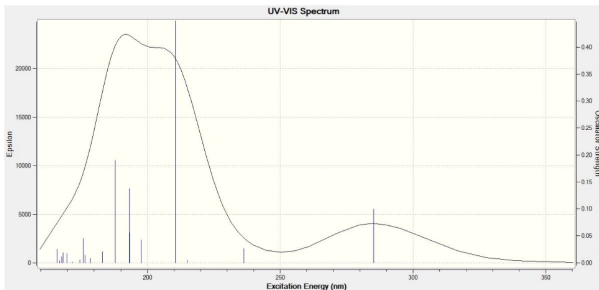
Slika 6.14: Apsorpcijski spektar prvog pobuđenog elektronskog stanja (ESA) molekule 3 dobiven TD-DFT računskom metodom.
