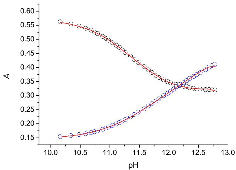
Slika 4.12 Usporedba izmjerenih ( \lambda = 462 nm ( \circ ), \lambda = 446 nm ( \circ )) i računanih (—) vrijednosti apsorbancije titracije na slici 4.10. Odabrane vrijednosti \lambda su maksimumi apsorbancije ne-deprotonirane i di-deprotonirane vrste prema modelu (4.16).
