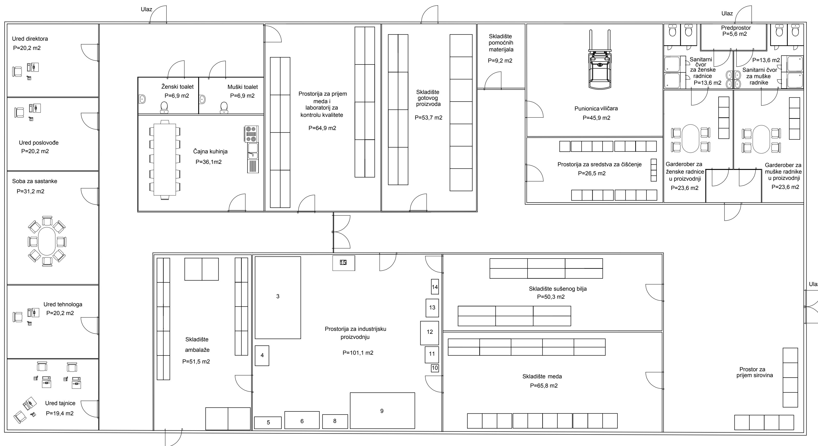
Slika 17. Tlocrt pogona za proizvodnju mješavine meda
