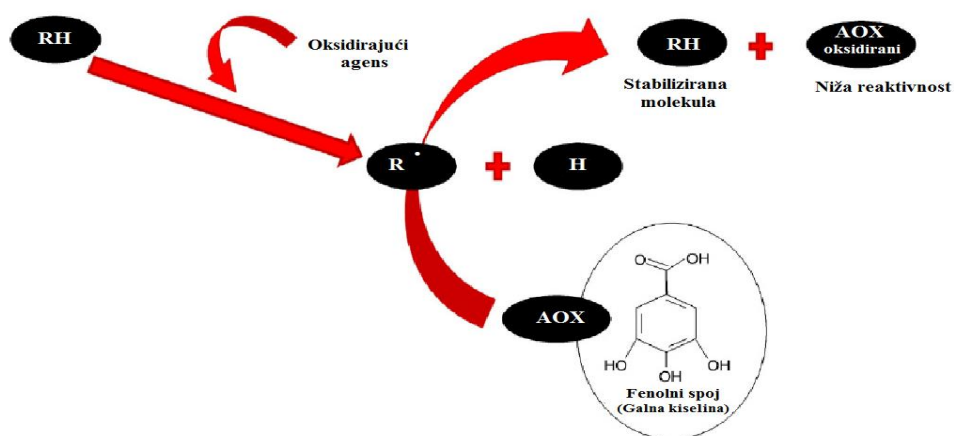
Slika 9. Mehanizam antioksidacijskog djelovanja fenolnih spojeva: AOX – antioksidans; R^\bullet – slobodni radikal, RH – molekula podložna oksidaciji (Wong-Paz i sur., 2017)
