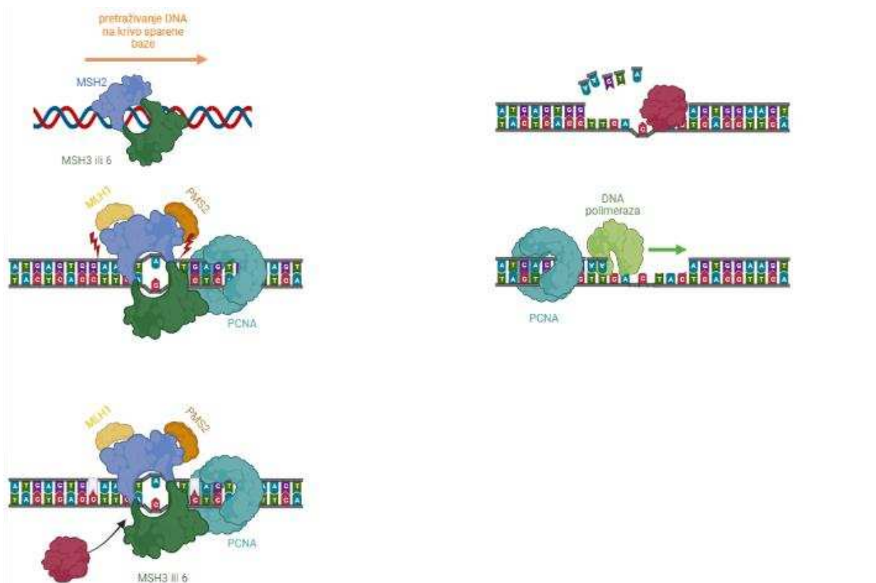
Slika 3. Prikaz sustava za popravak pogrešno sparenih baza. Dimer MSH2/MSH6 pretražuje dvostruku uzvojnicu na pogrešno sparene baze. Kad ih nađe, na MSH2/MSH6 dimer regrutiraju se MLH1 i PMS2 koji imaju endonukleaznu aktivnost. Nakon izrezivanja nukleotida oko pogrešno sparenih baza, egzonukleaza (EXO1) izreže dio lanca s pogrešno sparenom bazom i slijedi ponovna sinteza lanca DNA. PCNA, jezgrin antigen proliferirajuće stanice (naslikano u BioRenderu).
