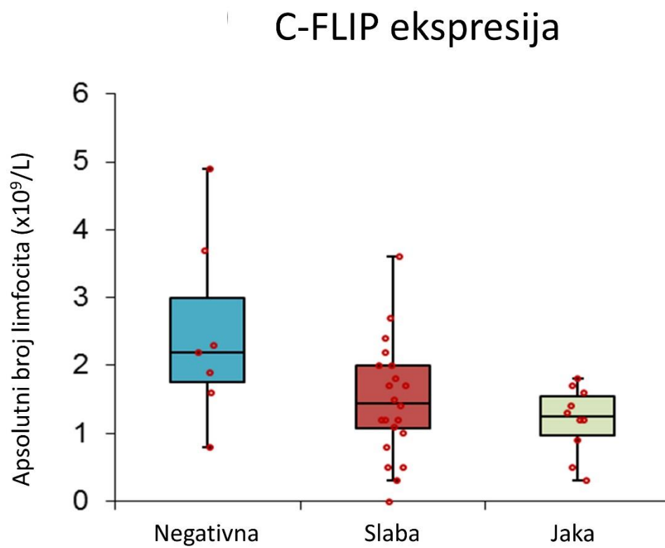
Slika 4: Negativna povezanost nižeg apsolutnog broja limfocita i ekspresije c-FLIP.
