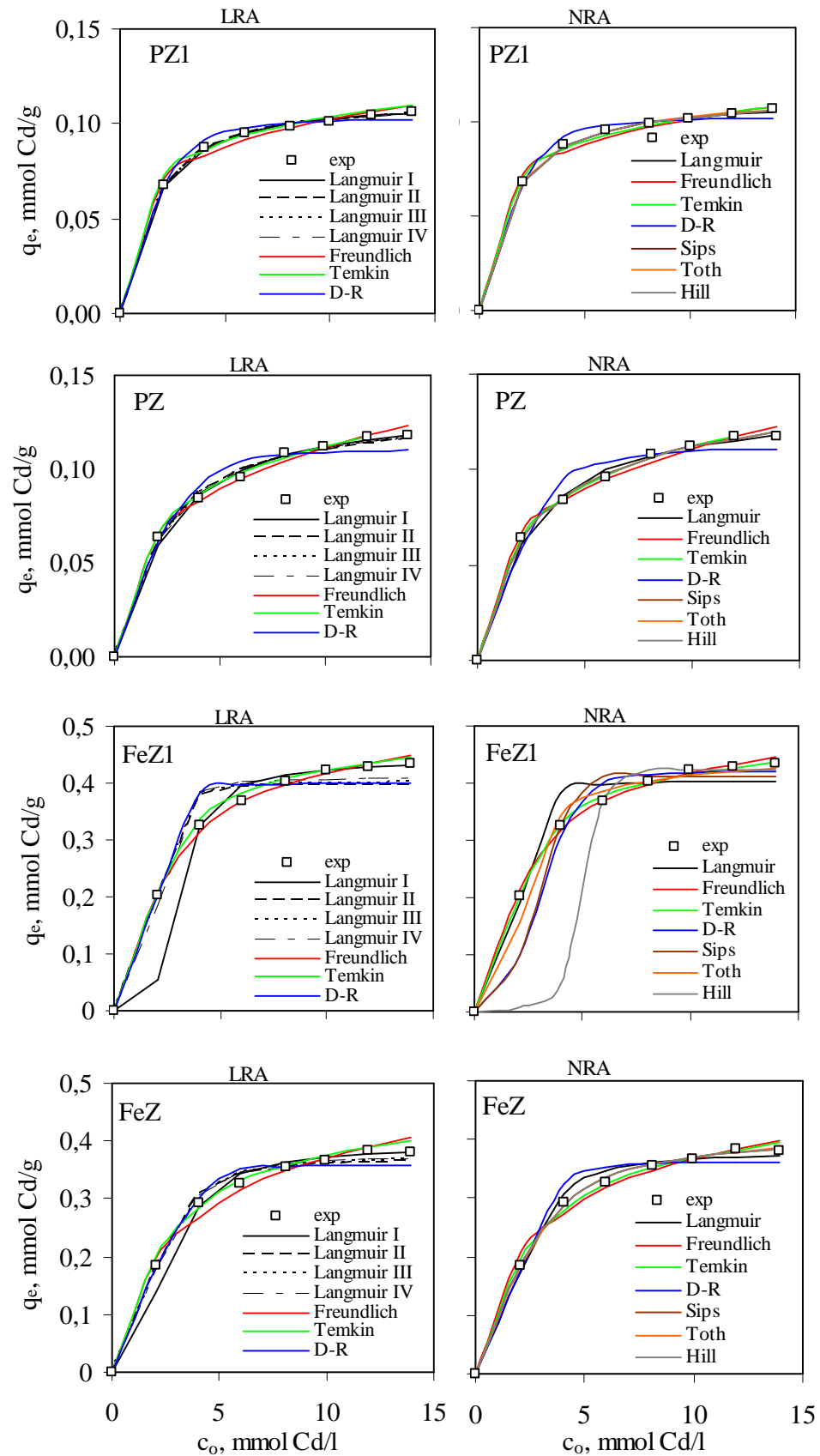
Slika 5.21. Usporedba ravnotežnih rezultata za vezivanje kadmija na PZ1, PZ, FeZ1 i FeZ s modelima izoterma primjenom linearne (LRA) i nelinearne (NRA) regresijske analize.
