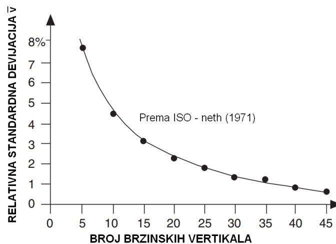
Slika 3.13 Broj brzinskih vertikalala u odnosu na točnost mjerenja srednje brzine
