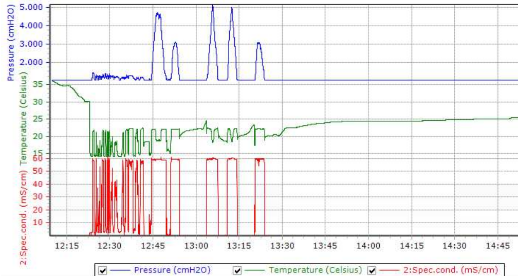
Slika 1.11 Prikaz učitanih podataka s CTD divera prilikom uzdužnog profiliranja rijeke cetine na ušću
