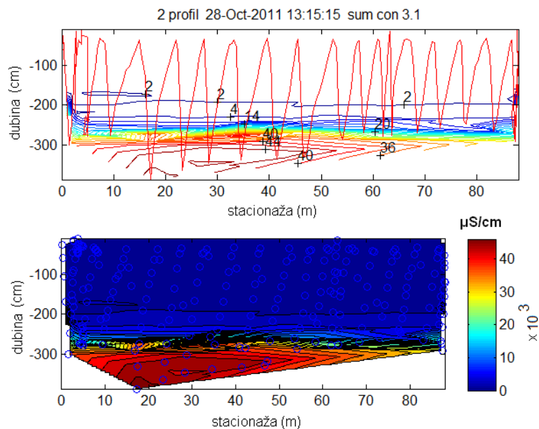
Slika 1.12 Raspodjela električne vodljivosti na poprečnom profilu rijeke Cetine, nedaleko od ušća
