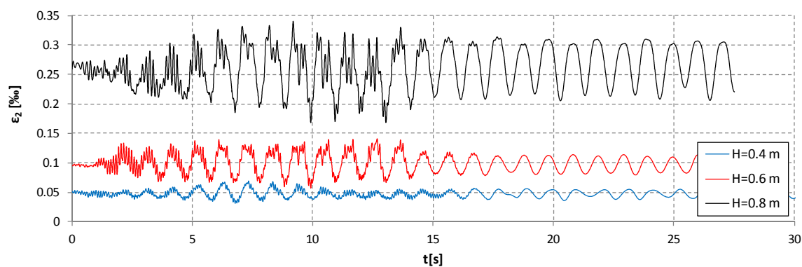
(b) Deformacija \varepsilon_2
