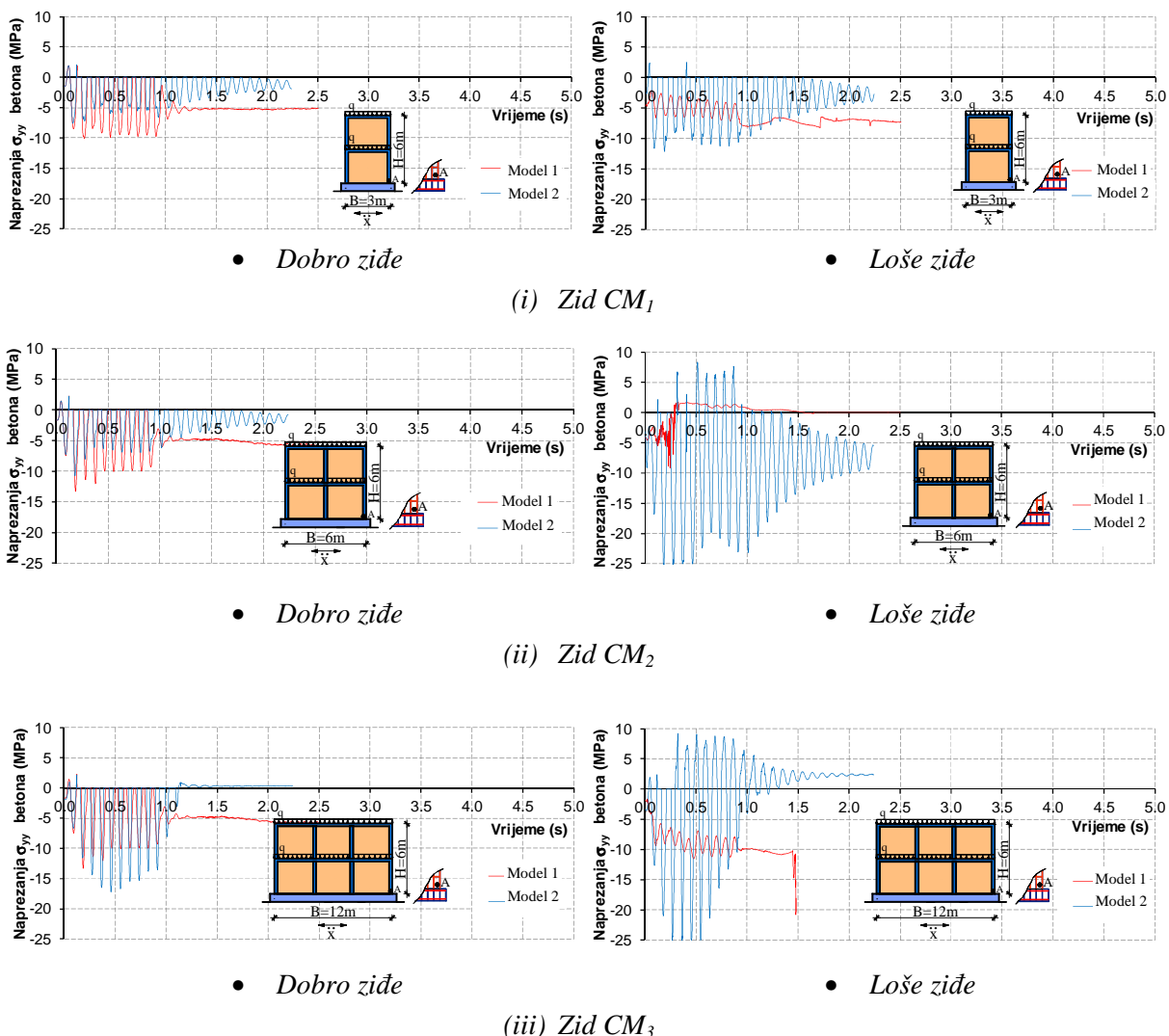
Slika 5.217. Vertikalno naprezanje u betonu u točki A omeđenih zidanih zidova izloženih harmonijskom ubrzanju podloge s a_{\max}=0,3g
