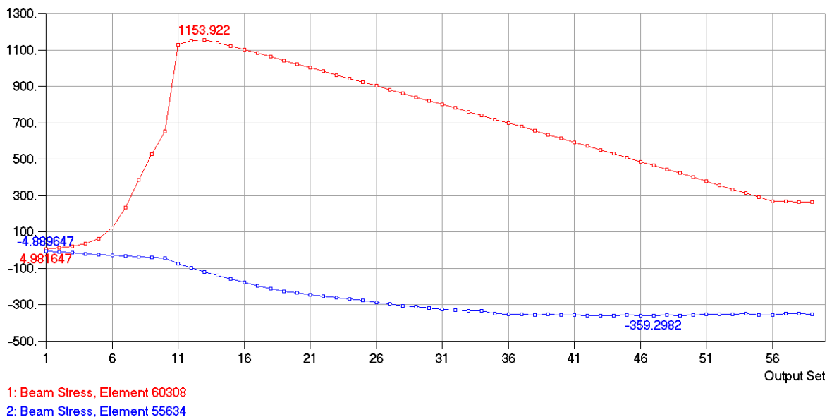
Slika 5.13. Najveća i najmanja napreznja u vlaknima za model M2_05
