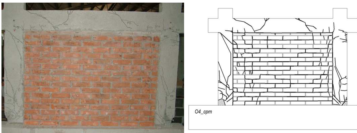
Slika 6.137 Prikaz oštećenja i pukotina ispitnog uzorka O4_cpm
