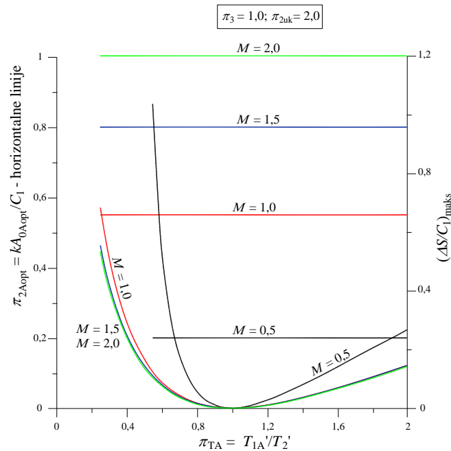
Slika 89. Zavisnost maksimalne generirane entropije (\Delta S/C_1)_{\text{maks}} i \pi_{2Aopt} umreženog rekuperatora o M i \pi_{TA} uz \pi_3 = 1,0 ; \pi_{2uk} = 2,0
