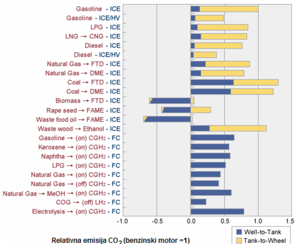
Slika 7.4. Relativna emisija CO 2 - izračun emisija stakleničkih plinova Well-to-Wheel analizom
