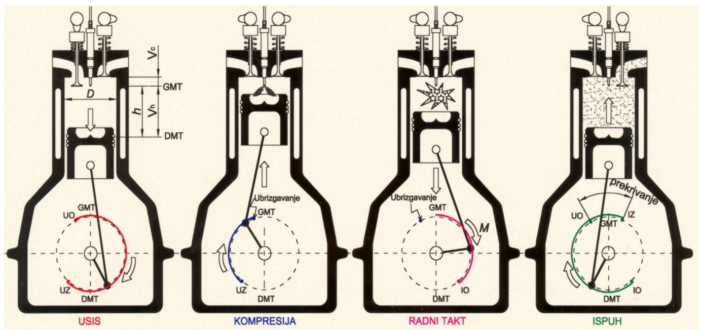
Slika 2.1. Shema rada četverotaktnog motora
