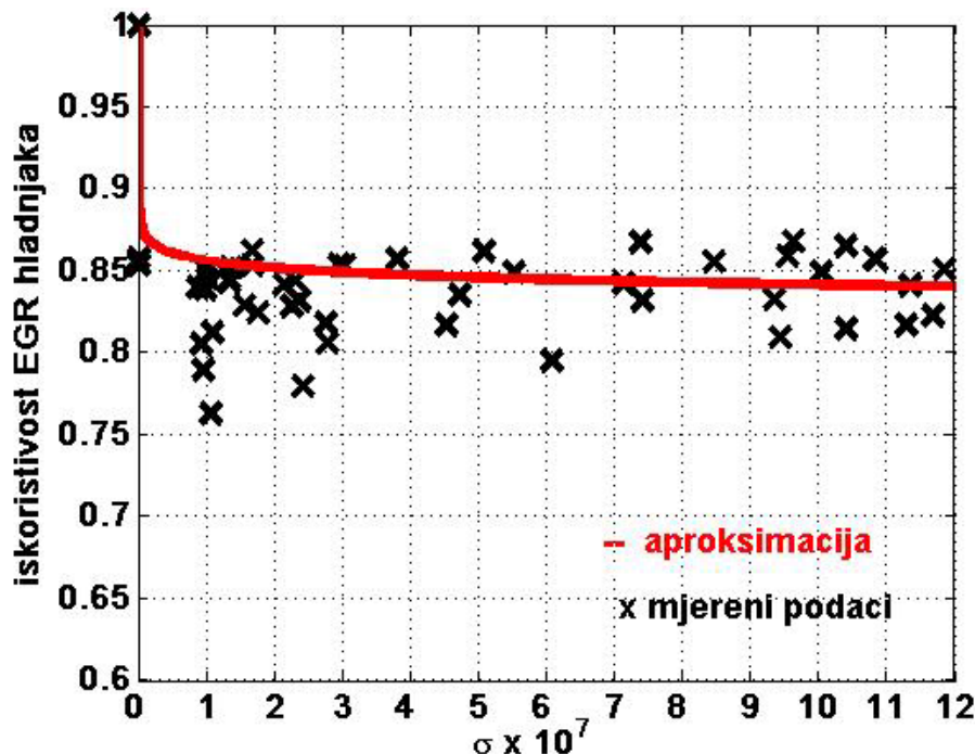
Sl. 4.17 Prikaz iskoristivosti topline EGR-hladnjaka u ovisnosti o parametru protoka dimnih plinova, \eta_{EGR} = f(\sigma) , [29] smatrati da je ova vrijednost približno konstantna, kao što se to može uočiti na slici 4.17. Temperatura ohlađenih dimnih plinova T_{6'} na izlazu iz EGR-hladnjaka računa se pomoću izraza:
