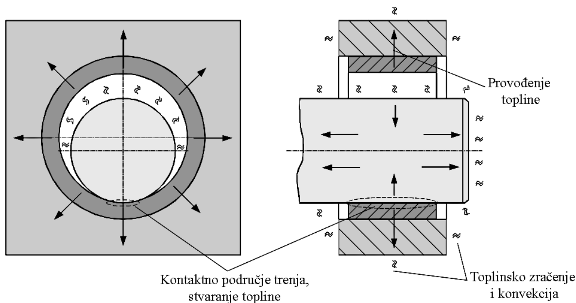
Slika 29. Stvaranje topline u sustavu klizni ležaj/rukavac
