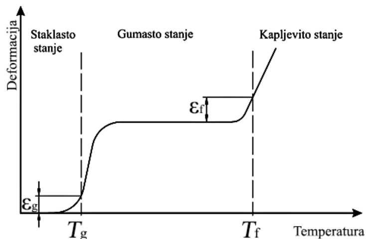
Slika 25. Termomehanička krivulja [25]
