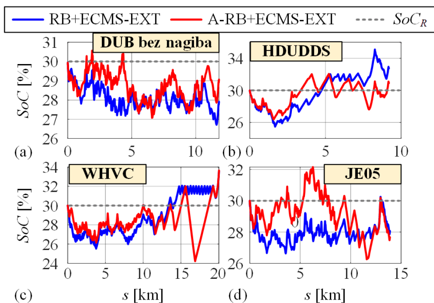
Slika 6-10. Usporedni odzivi SoC-a po prijeđenome putu dobiveni simulacijom A-RB+ECMS-EXT i RB+ECMS-EXT sustava upravljanja (FWD model i CS režim rada).
